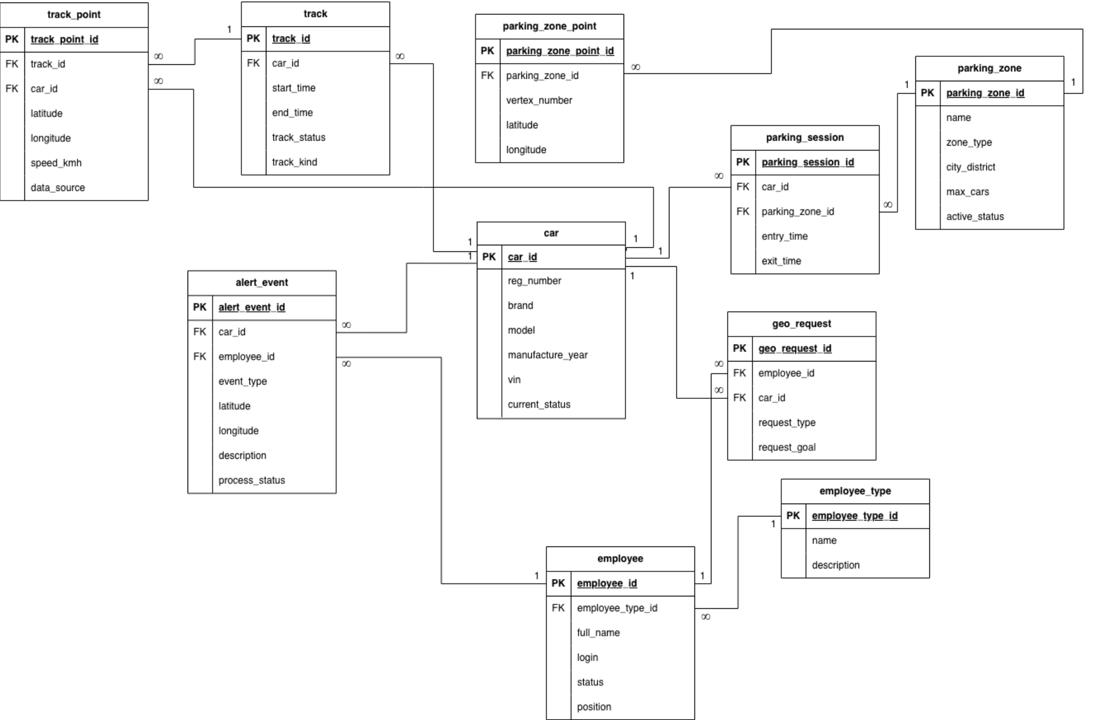
Рис. 4: Графическое описание схемы базы данных на английском языке
