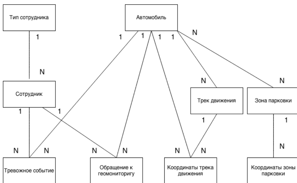
Рис. 2: Схема связи объектов предметной области
