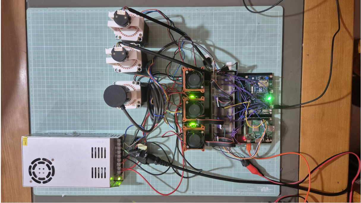
Figura 3.7: Protótipo do controlador CNC montado em bancada, com fonte de alimentação, motores de passo, drivers TMC5160, placa STM32 e Raspberry Pi.
