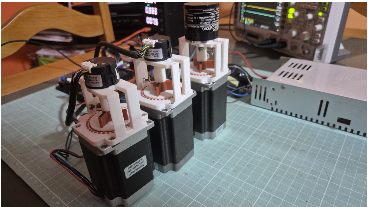
Figura 3.6: Vista dos motores de passo com suportes impressos em 3D, ponteiros e encoder TMCS-28 acoplado ao eixo para realimentação de posição.
