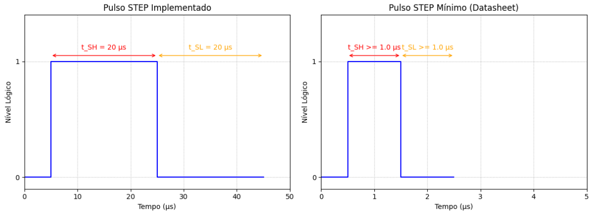
Figura 3.8: Comparação visual entre o pulso de STEP implementado no firmware (esquerda) e o pulso mínimo requerido pelo datasheet do TMC5160 (direita), evidenciando a robusta margem de tempo utilizada.
