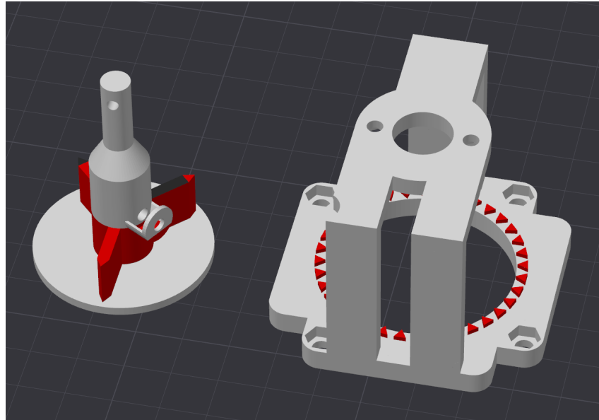
Figura 3.5: Modelo 3D do suporte do encoder TMCS-28 e do ponteiro acoplado ao eixo do motor de passo.
