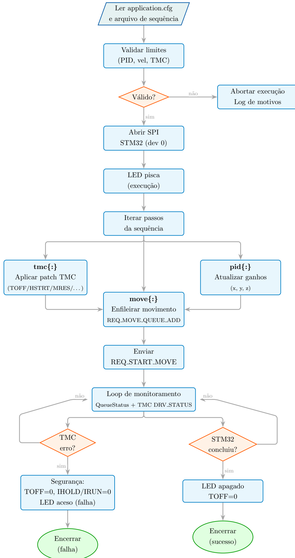
Figura 4.1: Fluxo do comando cnc-cli : validação, aplicação de patches TMC, enfileiramento de movimentos no STM32, monitoramento e estados do LED.
