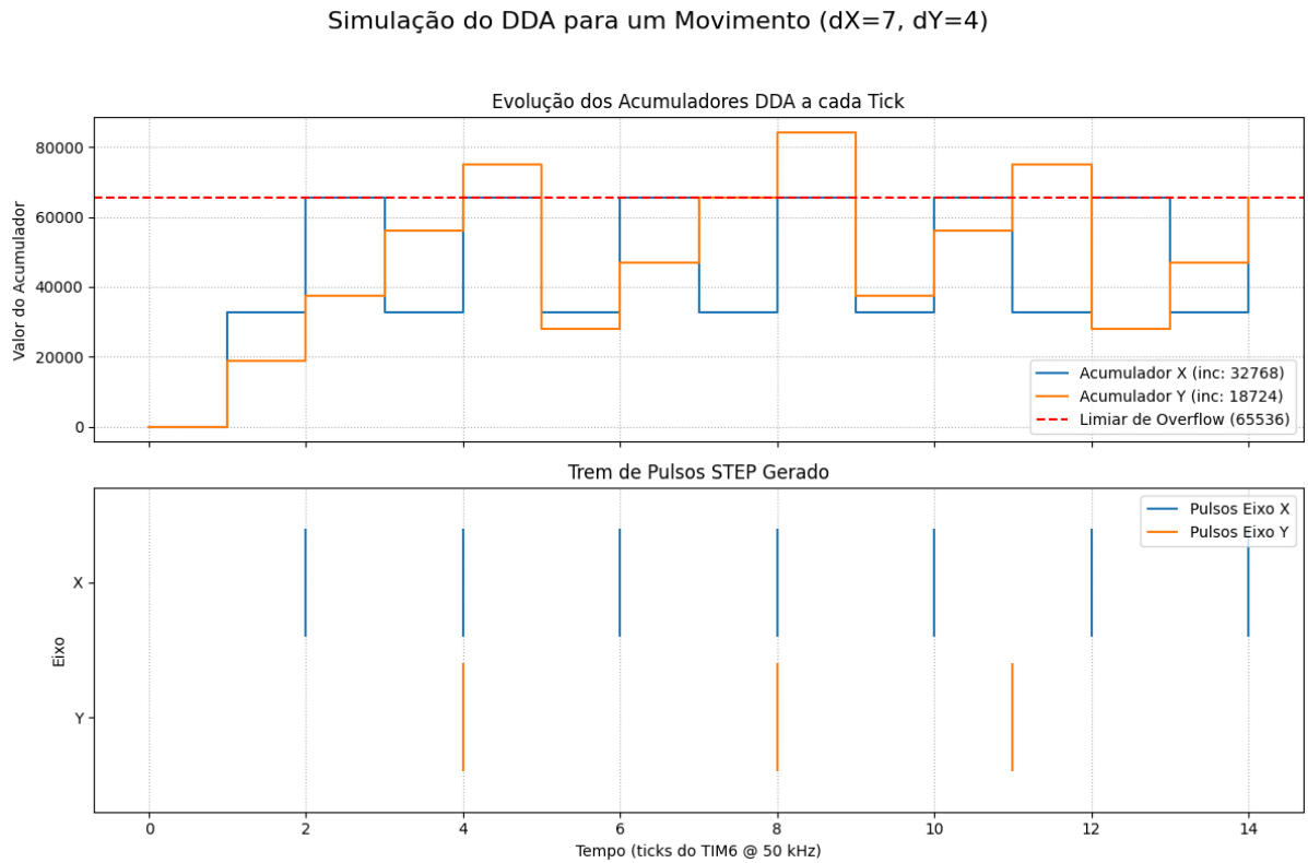
Figura 3.9: Simulação da operação interna do DDA para um movimento de 7 passos em X e 4 em Y. O gráfico superior mostra a evolução dos acumuladores de fase, e o inferior mostra os pulsos STEP gerados para cada eixo a cada transbordamento.
