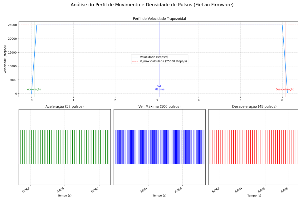
Figura 3.10: Perfil de velocidade da rampa trapezoidal simulado a partir dos parâmetros do firmware.
