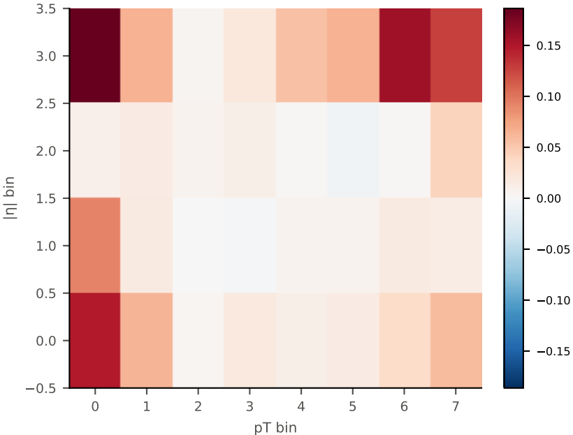
(d) where flat transport fails, all jets (1e-3 nats/jet) excess 1.26 \pm 0.04 , z 30.6
