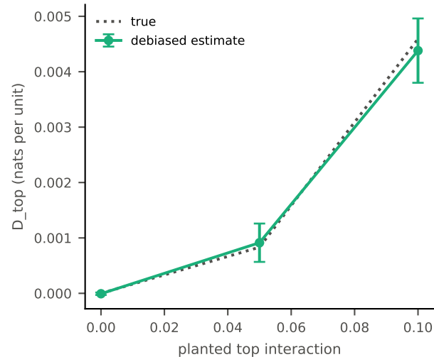
(d) order-4 information
