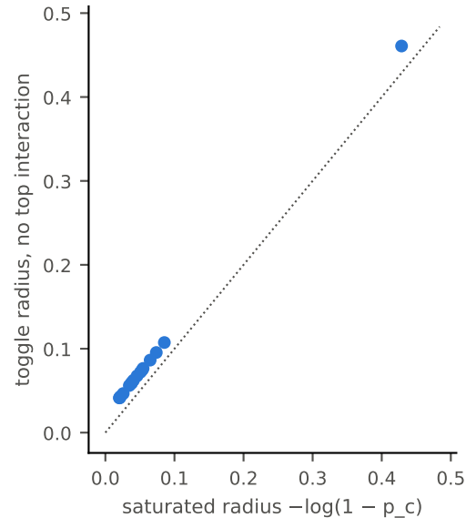
(d) [S] toggle radius (MBIC 4)
