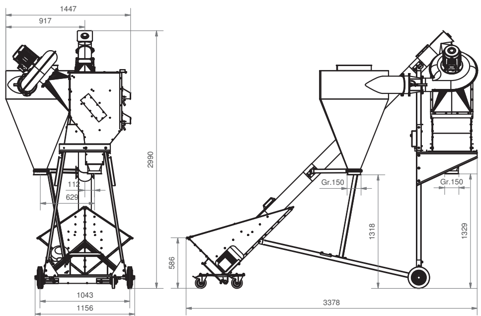
Maße Typ AR 25
