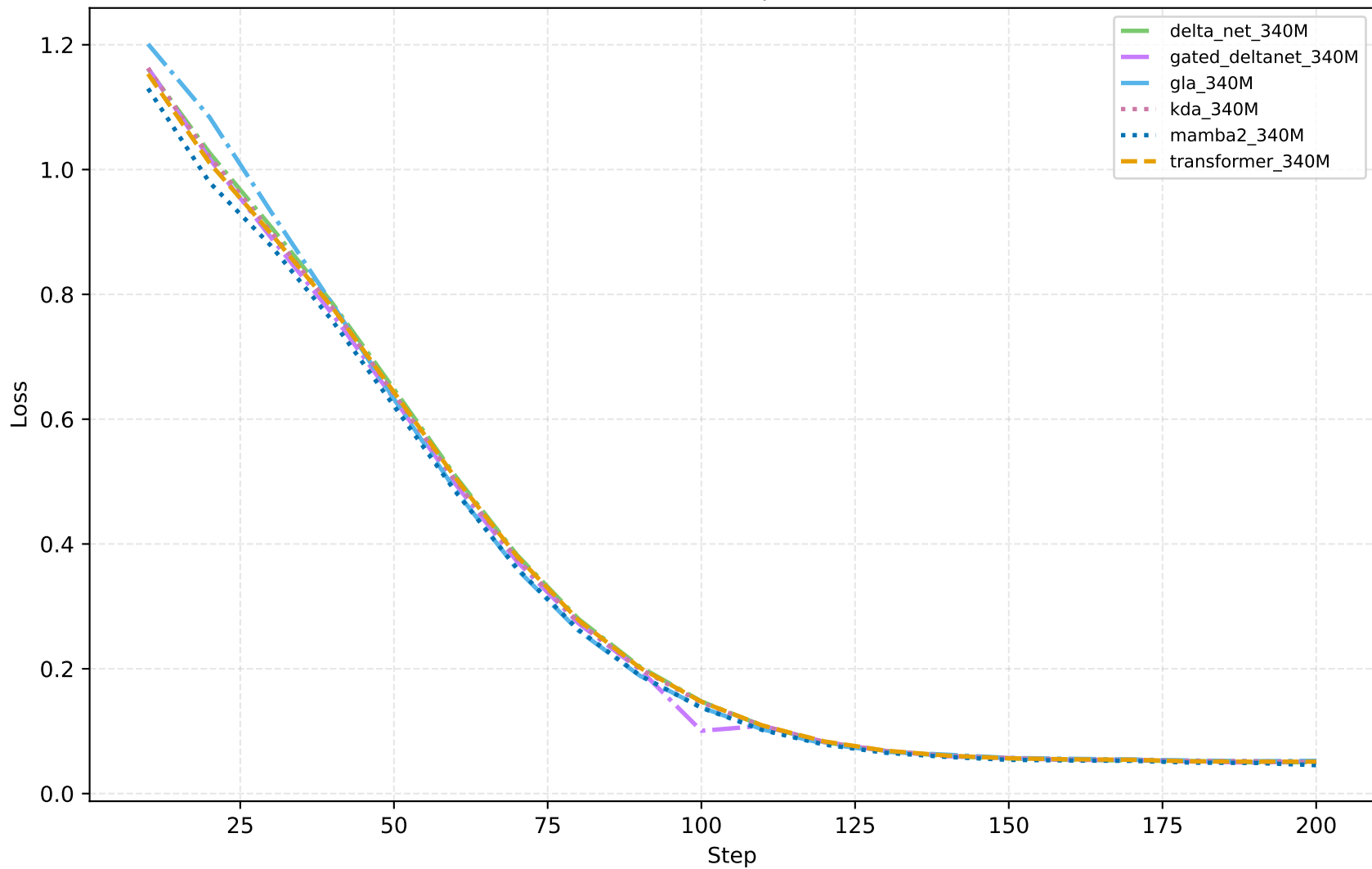
Eval Loss (Steps 1-200)
