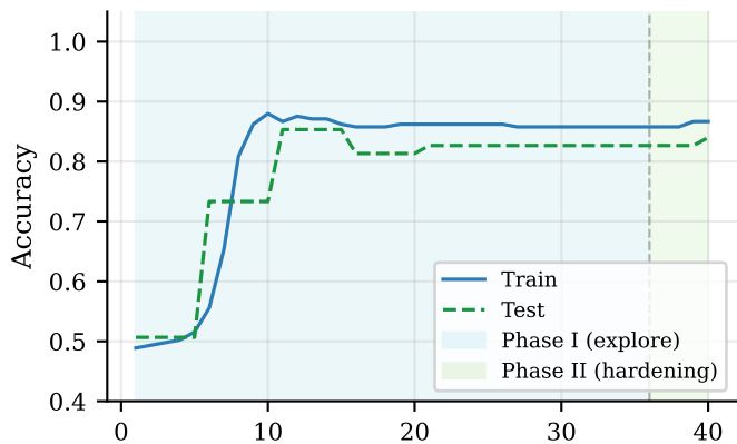
(d) MNIST 0 vs 1: Classification accuracy
