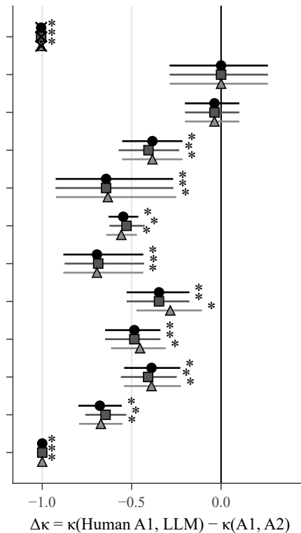
Qwen3 8B
