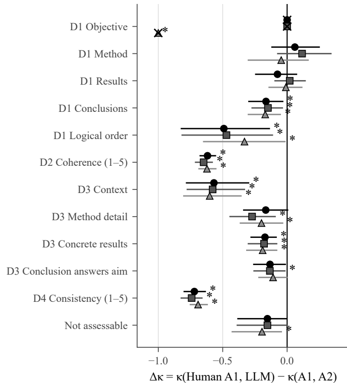
gpt-oss-20B
