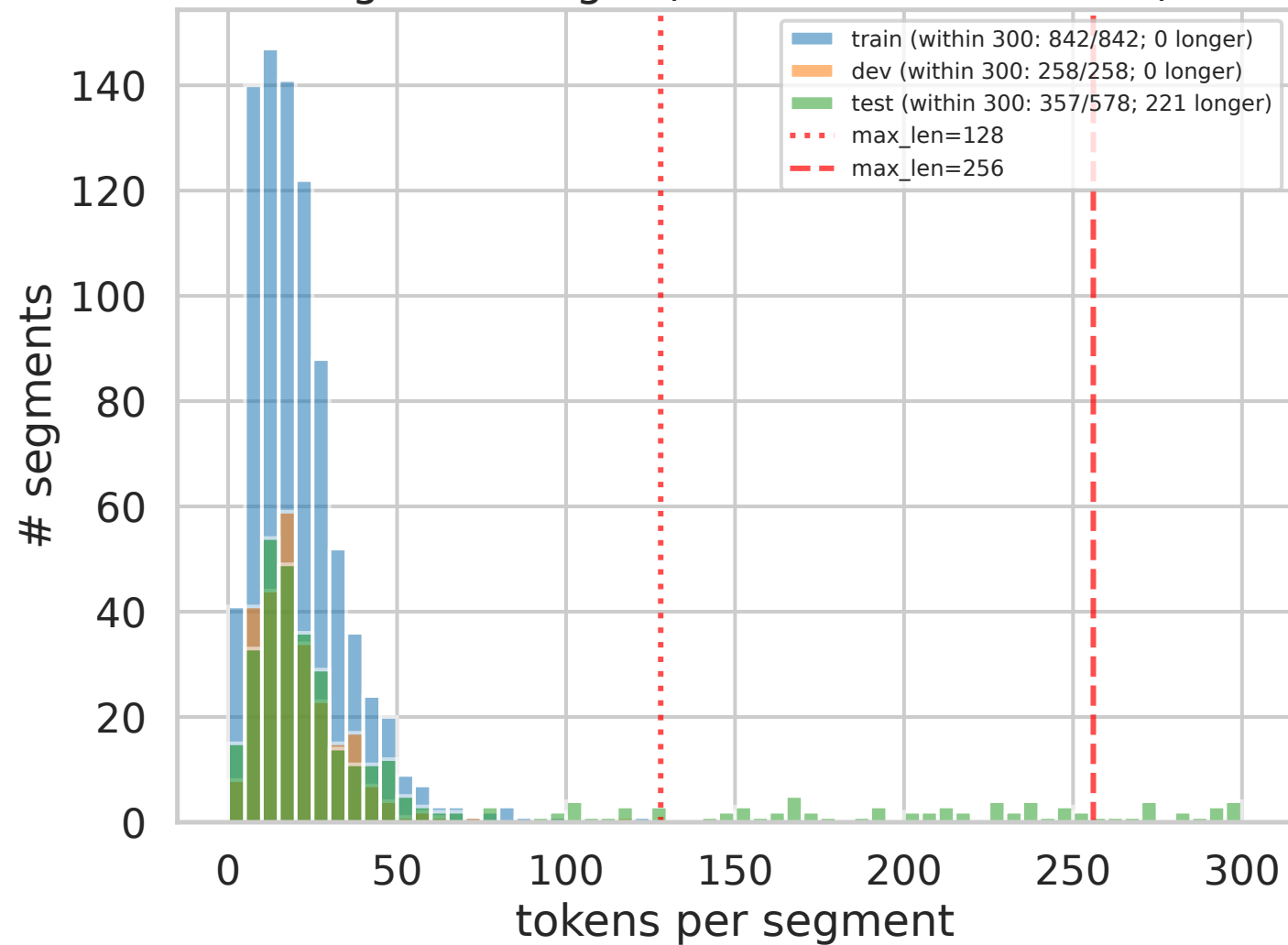
Segment length (zoomed 0-300 tokens)
