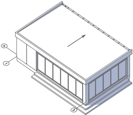
Аксонометрия крыши
