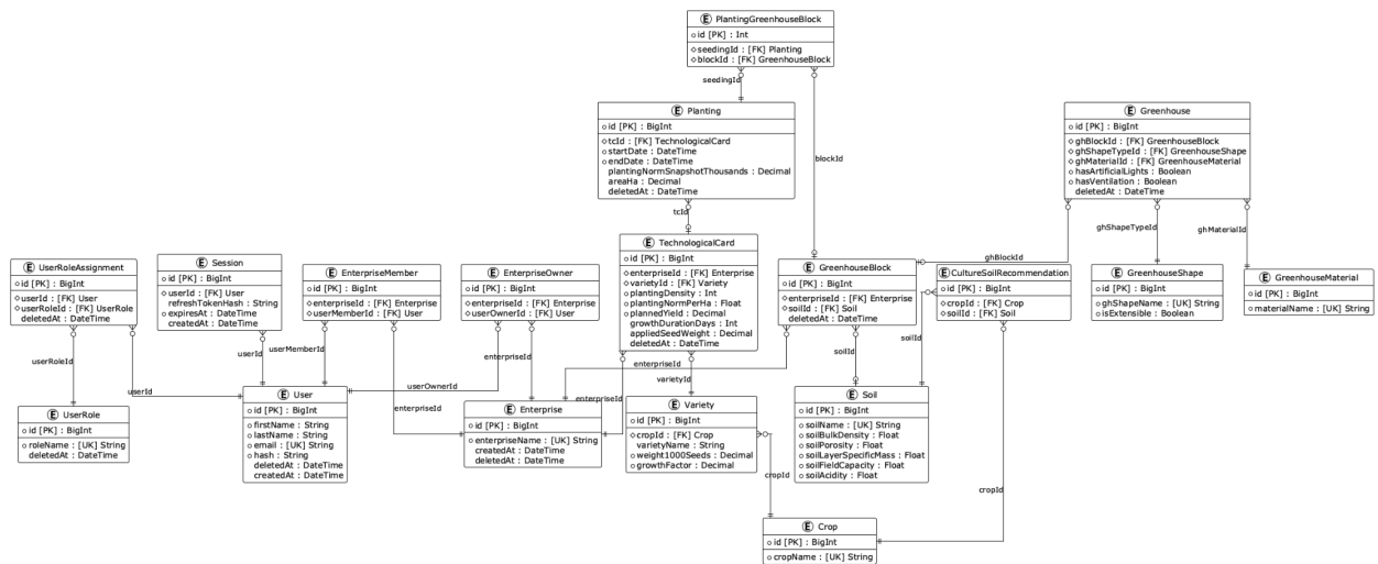
Рисунок 2.2.2.1 — ER-диаграмма БД
