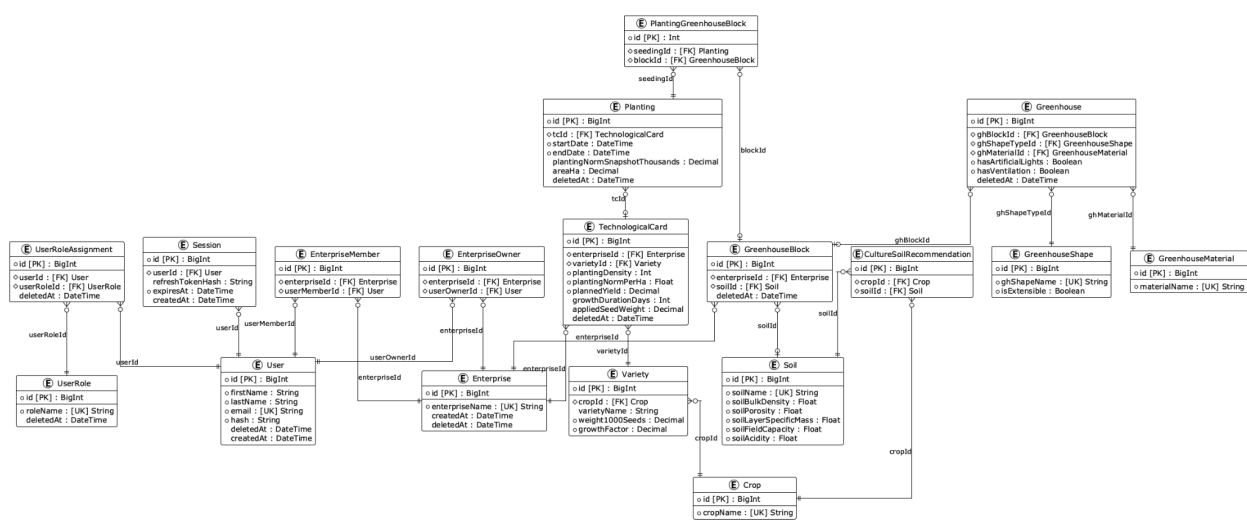
Рисунок 2.2.2.1 — ER-диаграмма БД
