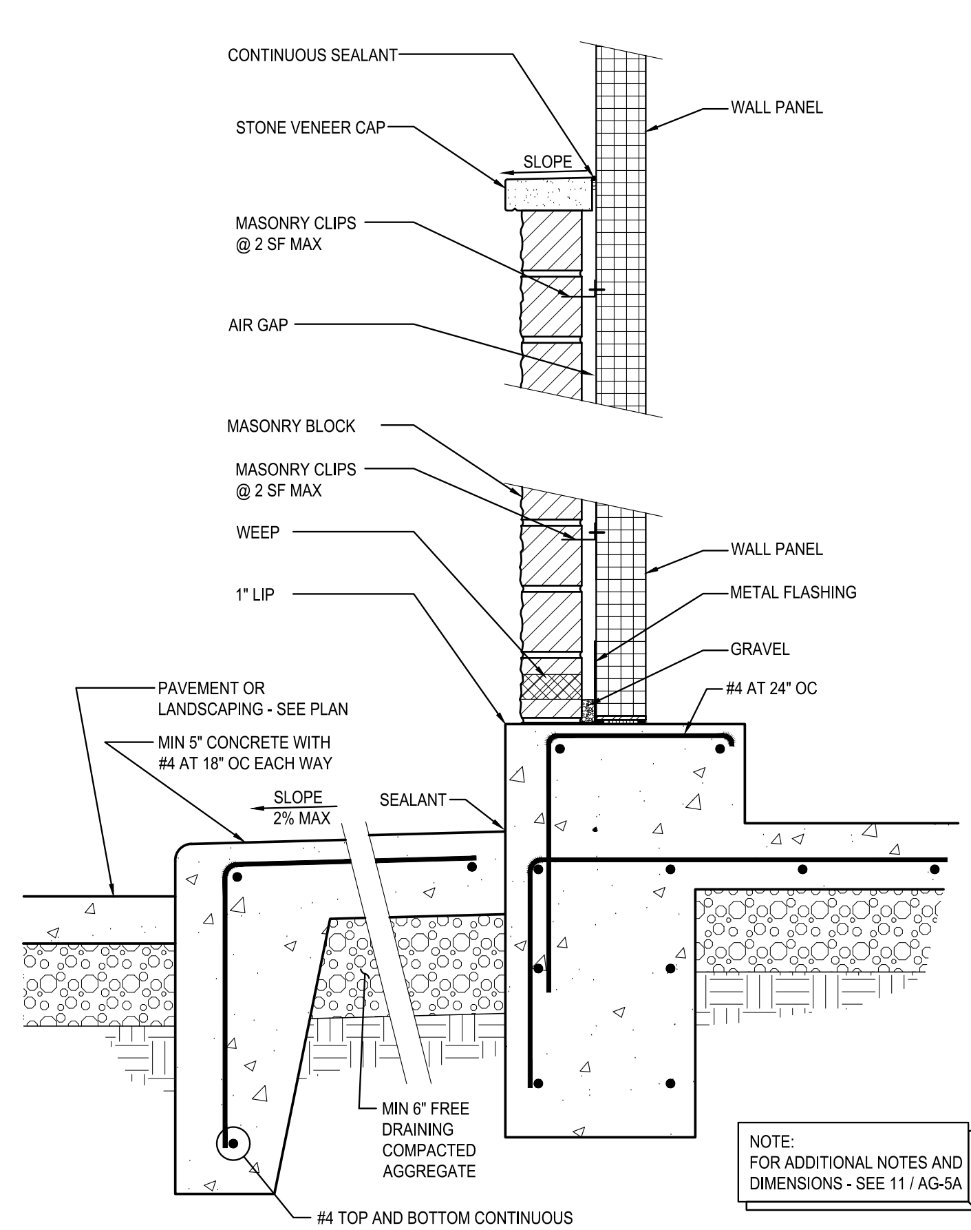
6 TYPICAL EDGE OF WALK SCALE: 1-1/2" = 1'-0" 1021
