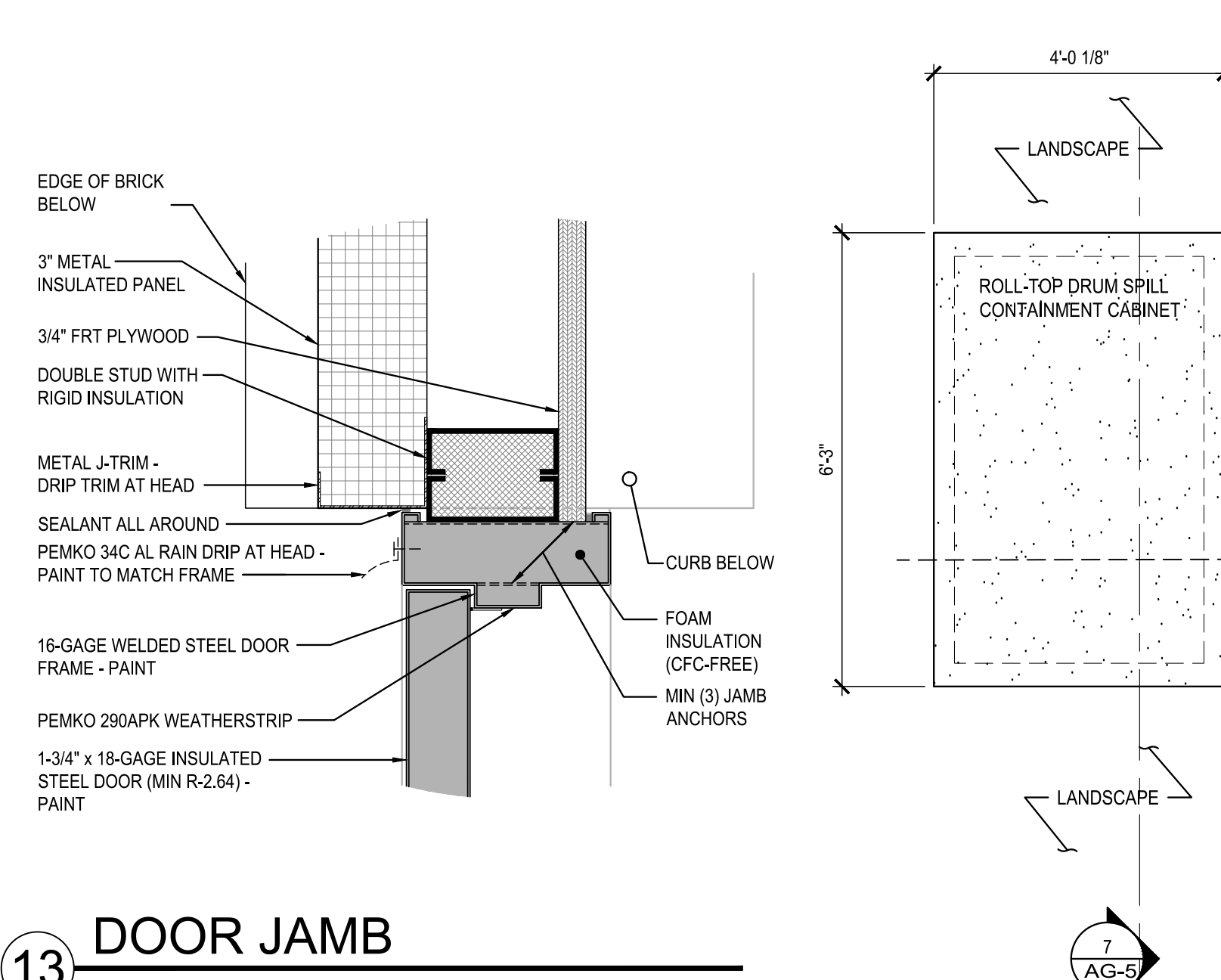
13 DOOR JAMB SCALE: 3" = 1'-0" (HEAD SIMILAR) 0122
