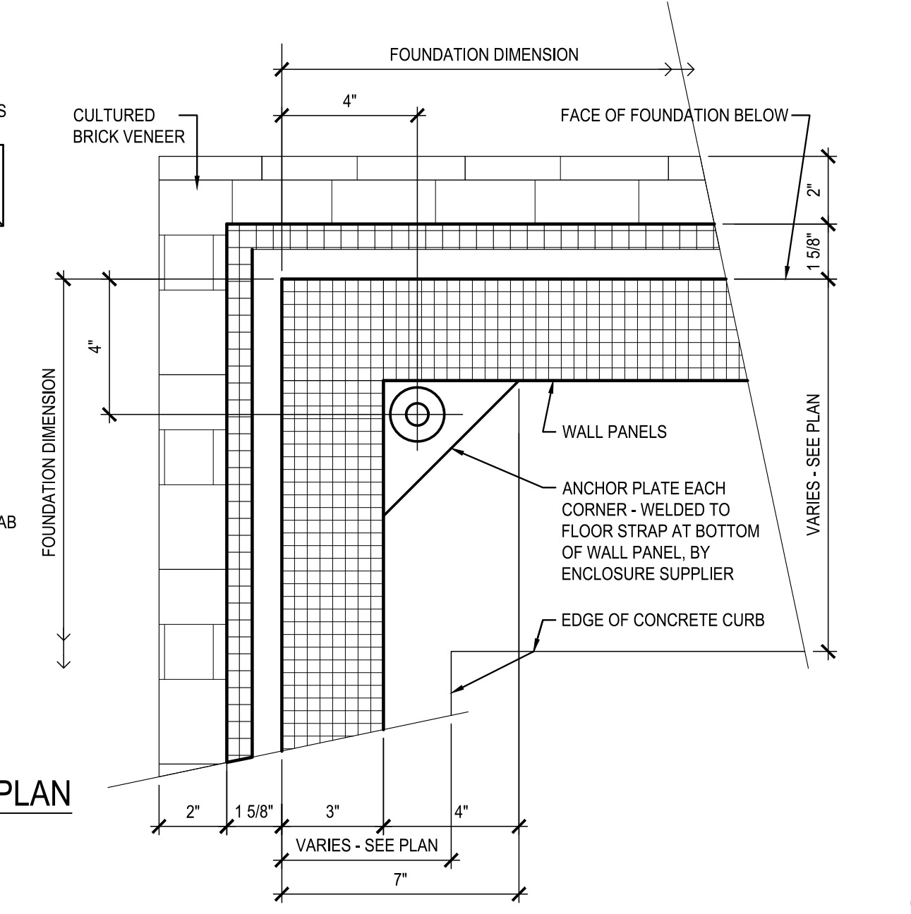
17 FOUNDATION CORNER SCALE: 3" = 1'-0" 0421
