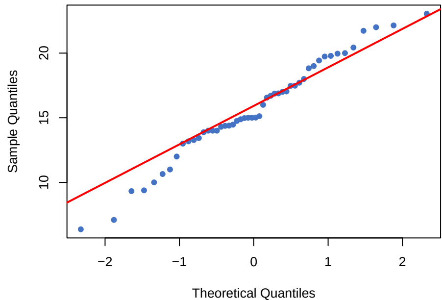
Gráfica QQ-Normal
