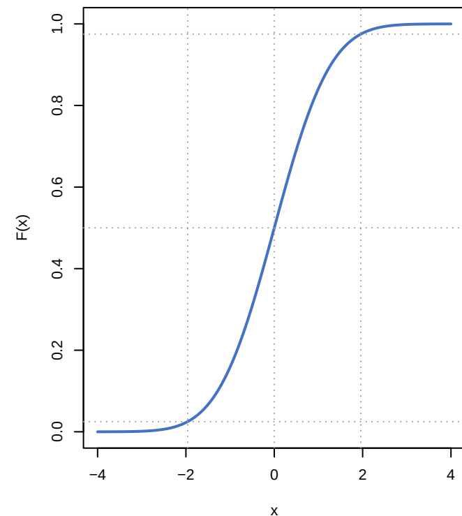
FDA — Normal(0,1)
