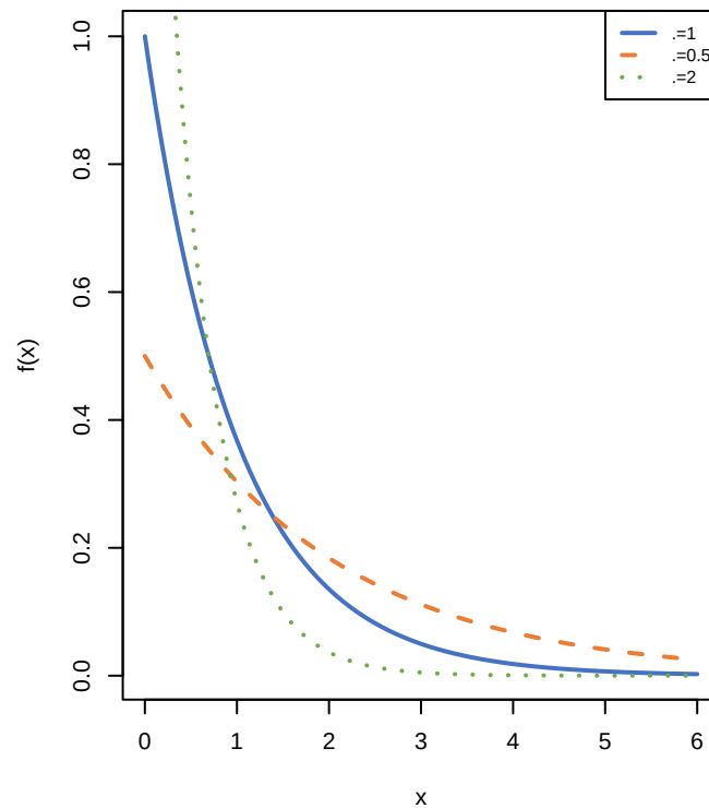
Exponential(.)
