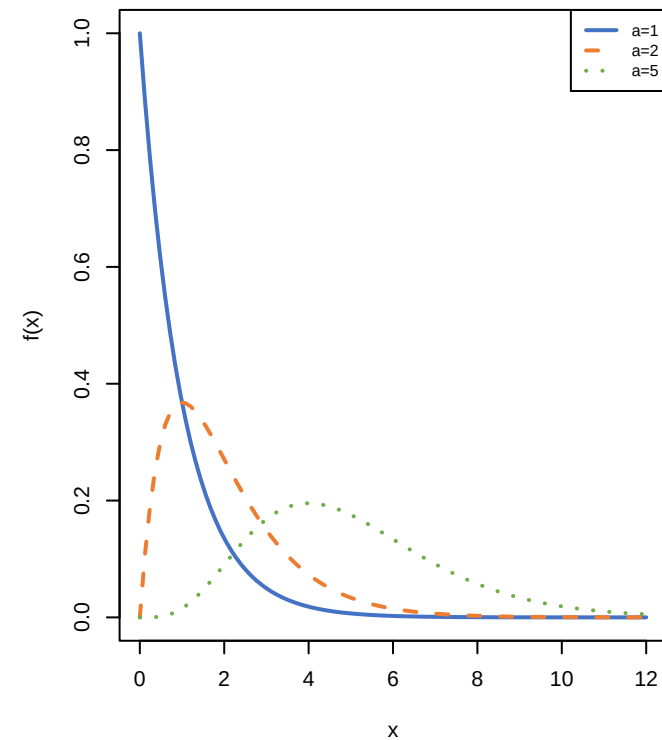
Gamma( a , 1)
