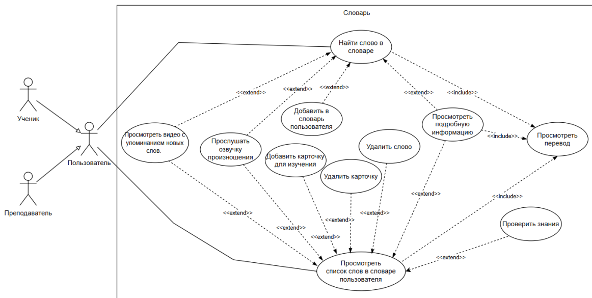
Рисунок 2. Диаграмма Use Case для версии 2.0 веб-приложения Chatty
