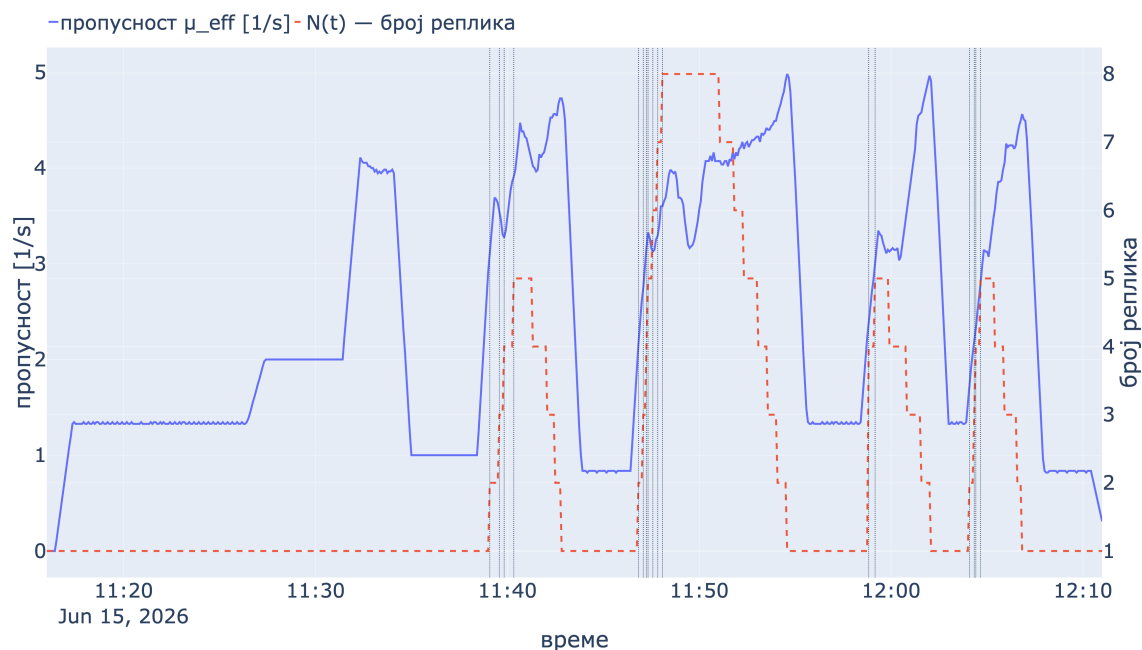
Слика 5.7: КЕДА - догађаји скалирања (испрекидане вертикалне линије) и пропусност у времену - план са наглим скоковима оптерећења.
