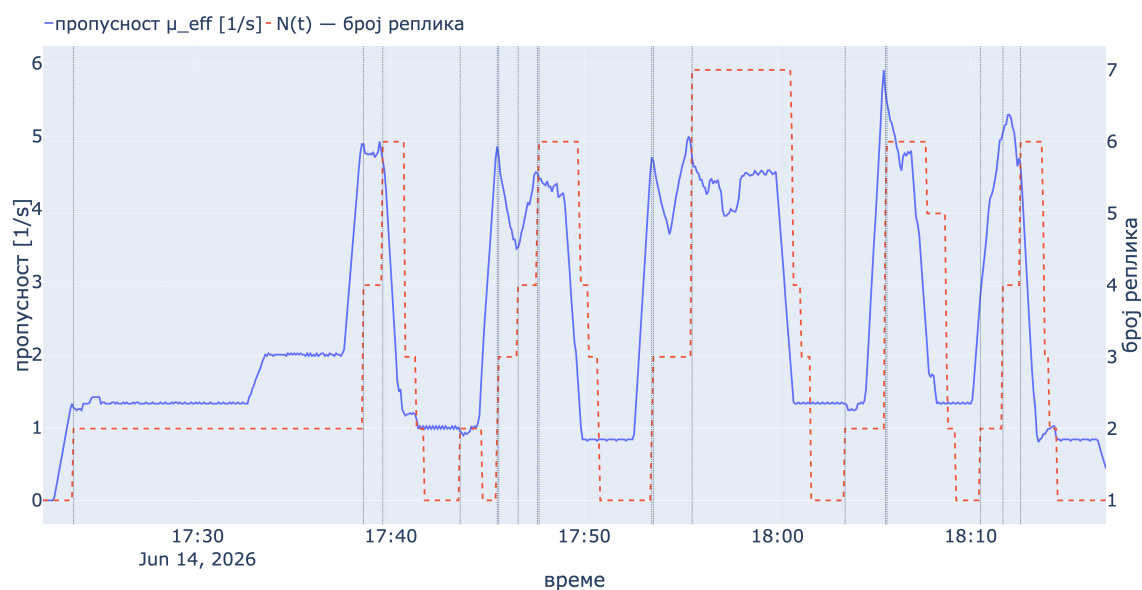
Слика 5.8: ХАСП - догађаји скалирања (испрекидане вертикалне линије) и пропусност у времену - план са наглим скоковима оптерећења.
