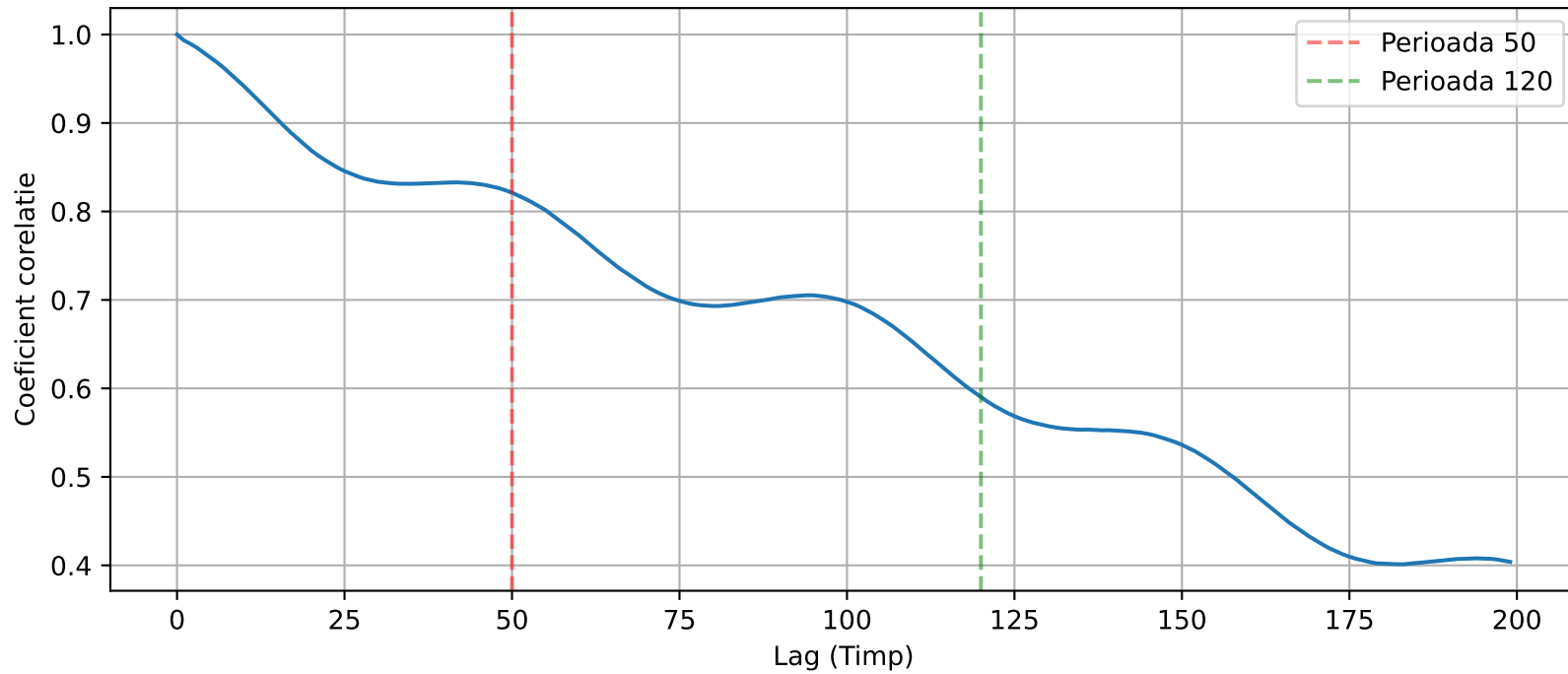
Autocorelatie (Primele 200 lag-uri)
