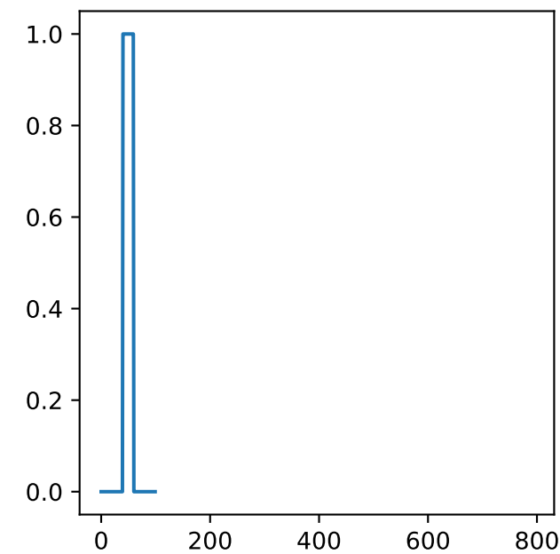
x[n] Bloc
