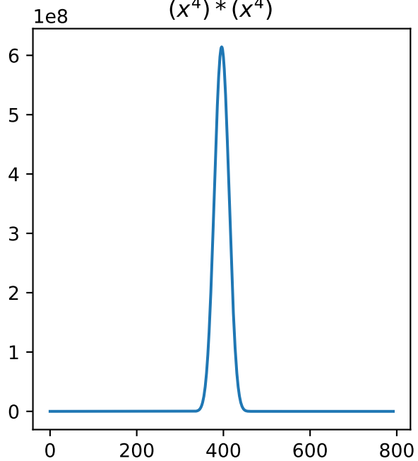
(x^4) * (x^4)
