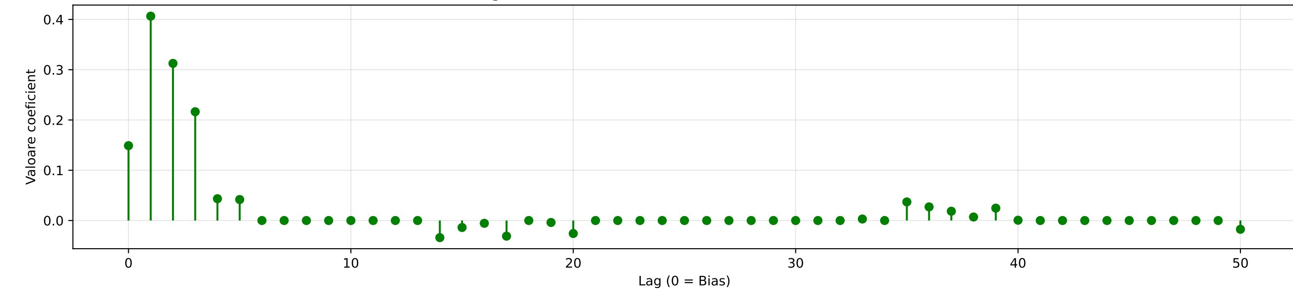
Regularizare L1 (lambda=250 -&gt; 20 coeficienti nenuli)
