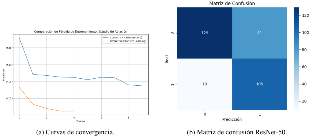
Figura 1: Comparación cuantitativa del entrenamiento y evaluación de los clasificadores de texturas.
