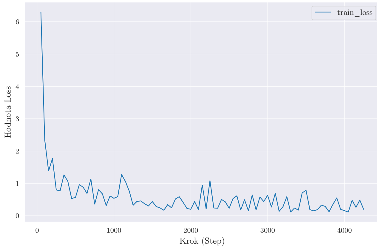
Průběh Loss ('train_loss') během trénování
