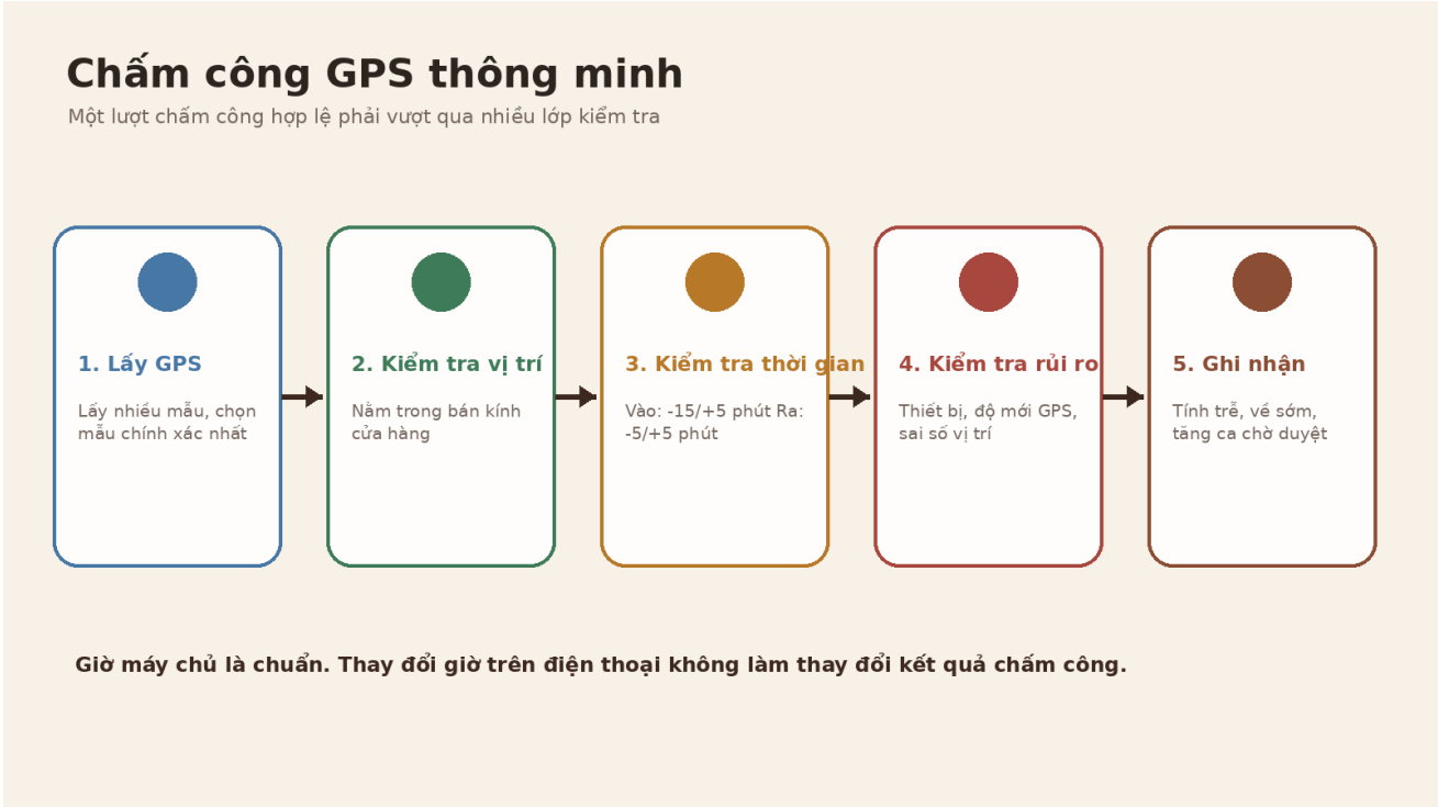
Hình 9. Các lớp kiểm tra chấm công
