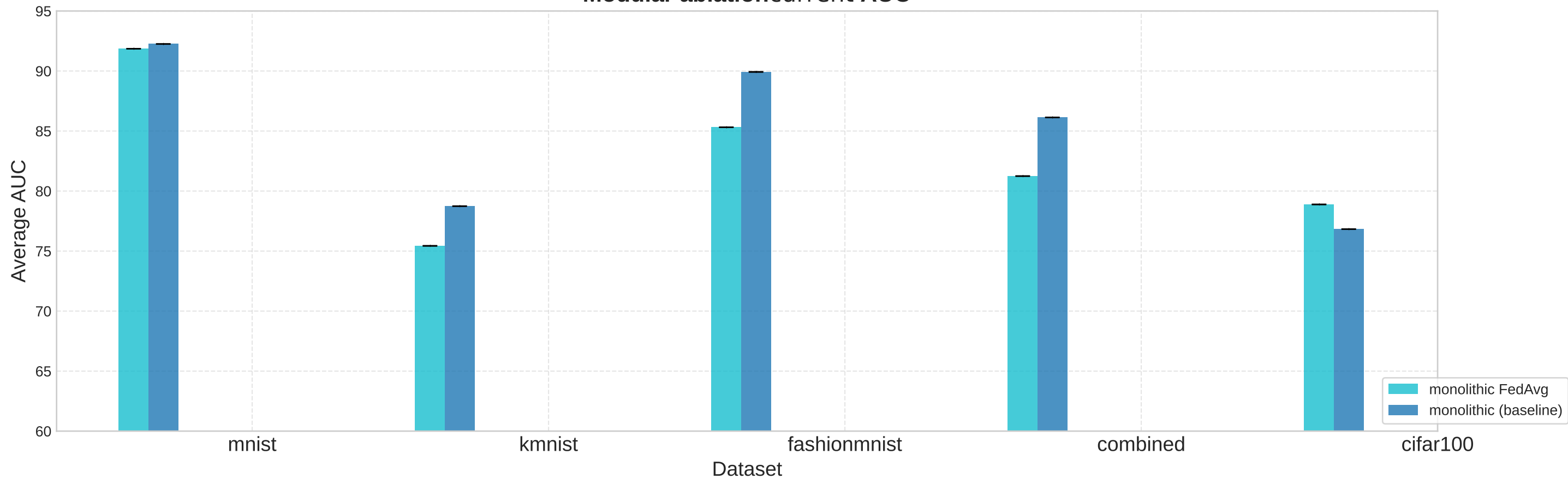
Modular ablationcurrent AUC
