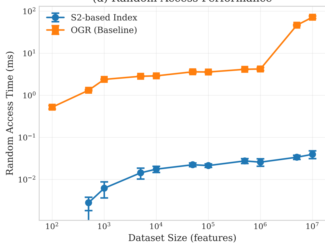
(d) Random Access Performance
