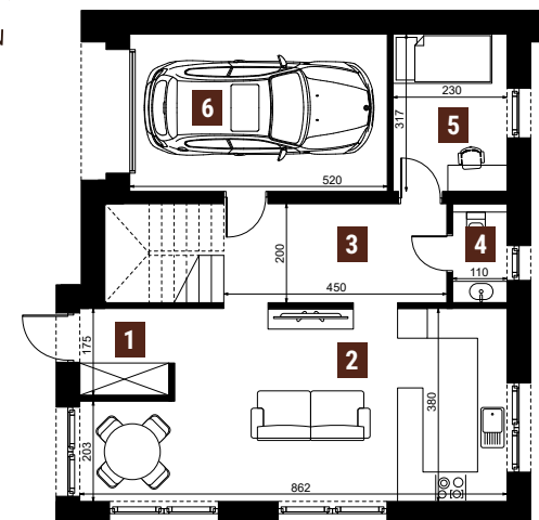
Rzut parteru
