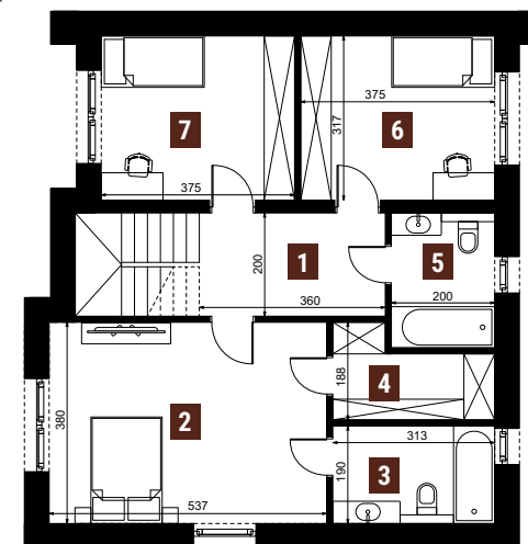
Rzut poddasza
