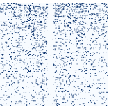
PR WT +ligand KLF motif
