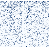
PR WT +ligand TEAD motif
