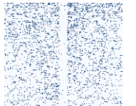
PR WT +ligand AP1 motif
