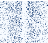
PR WT +ligand NR motif
