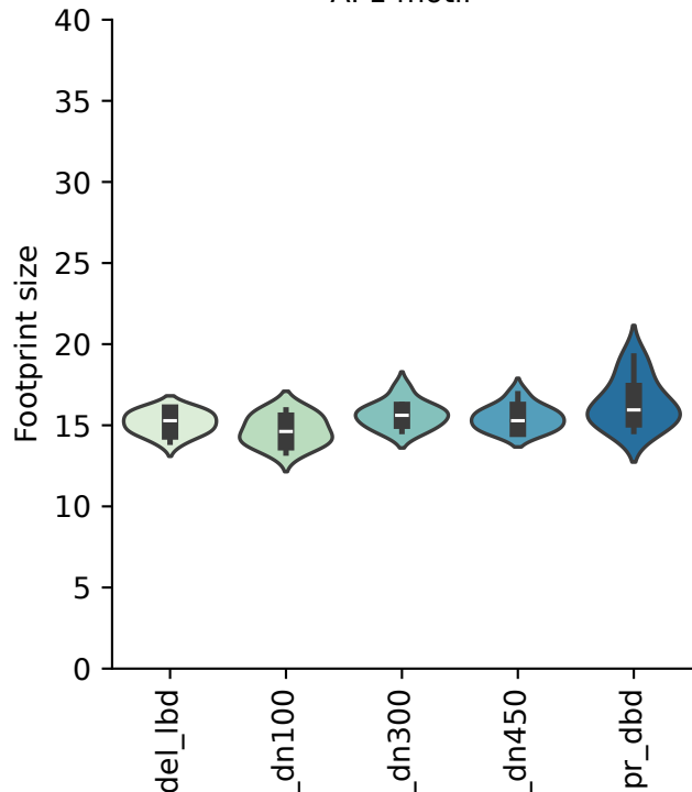
AP1 motif
