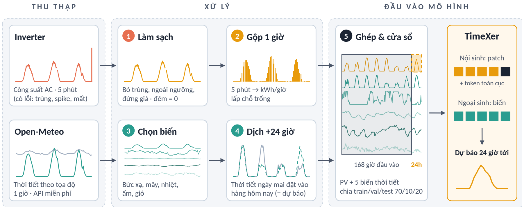
Hình 1. Luồng dữ liệu. Nhánh trên (cam): sản lượng PV từ inverter, là biến cần dự báo. Nhánh dưới (xanh): thời tiết, là biến hỗ trợ. Hai nhánh ghép theo giờ, cắt thành cửa sổ 168 giờ → 24 giờ cho TimeXer.
