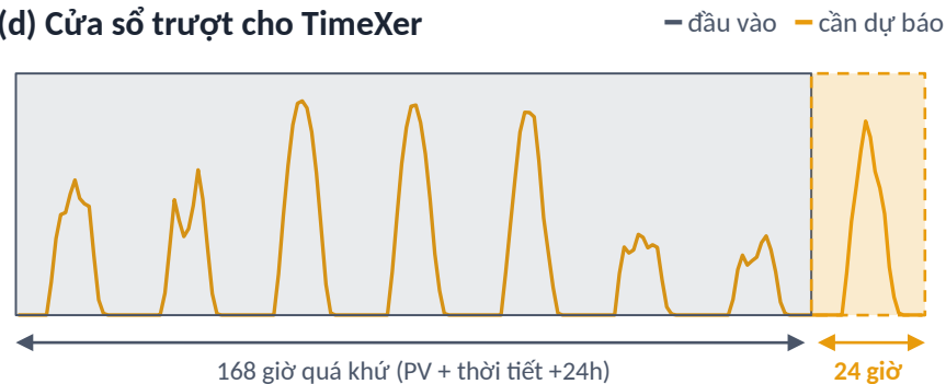
Hình 2. (a) Lọc điểm lỗi trong log inverter. (b) Gộp theo giờ; khoảng trống dài được ước lượng từ bức xạ. (c) Cột thời tiết dịch lên 24 giờ nên cửa sổ đầu vào chứa sẵn thời tiết ngày mai. (d) Mỗi mẫu: 168 giờ đầu vào → 24 giờ cần dự báo.
