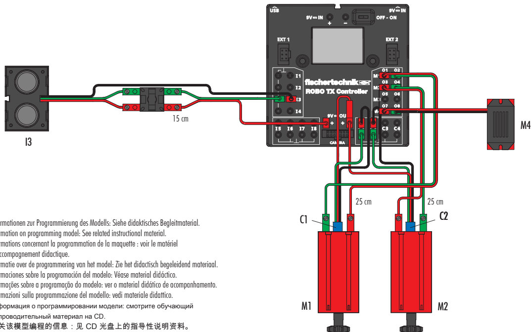
Schaltplan Circuit diagram Plan électrique
