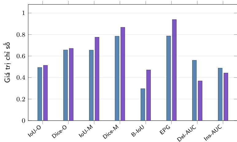
GlaS 2015
