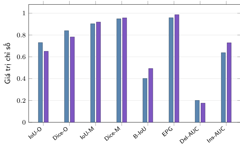
PH2
