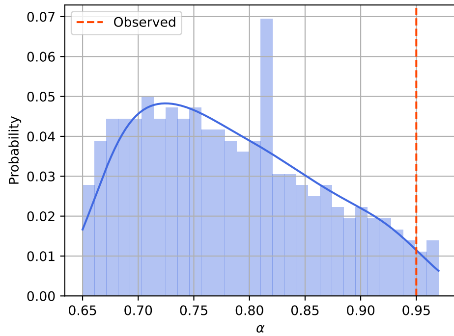
\alpha , posterior distribution
