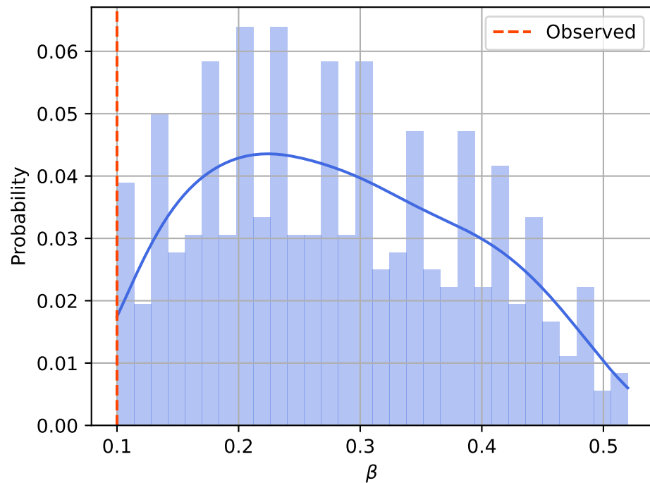
\beta , posterior distribution
