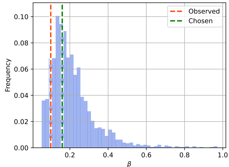
\beta , posterior distribution
