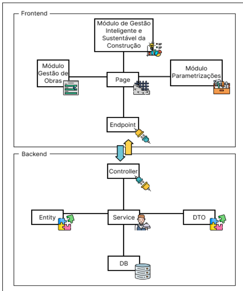
Figura 12: Arquitetura lógica da solução
