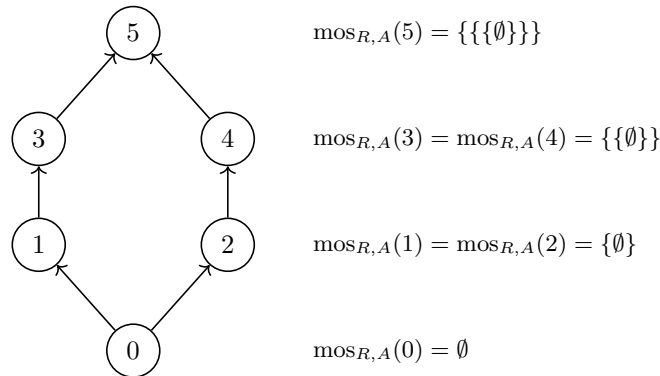
Figura 9.1: Diagrama de (A, R) no Exemplo 9.6.6.
