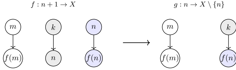
Figura 4.1: Subcaso k \neq n do Caso 2: a seta k \mapsto n é substituída por k \mapsto f(n) ; para m < n com m \neq k , continua valendo g(m) = f(m) .
