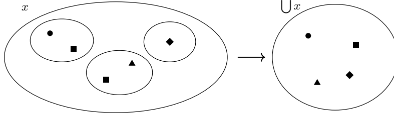
Figura 2.3: A união \bigcup x é o conjunto dos elementos de elementos de x .
