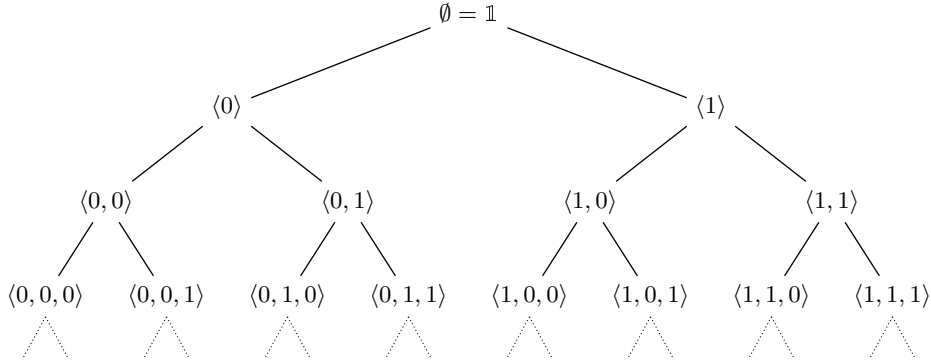
Figura 14.2: Os primeiros níveis de 2^{<\omega} .
