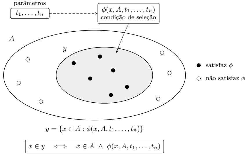
Figura 2.1: Compreensão como separação: a fórmula \phi , com parâmetros t_1, \dots, t_n , seleciona em A os elementos que formam y \subseteq A .
