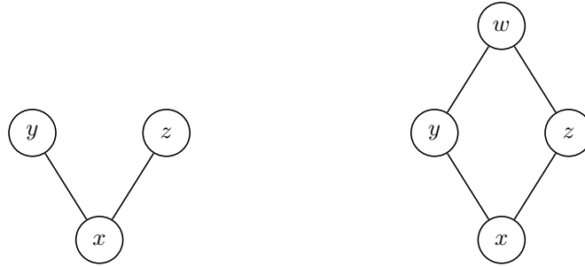
Figura 2.4: À esquerda, há elementos maximais sem elemento máximo. À direita, há um elemento máximo.
