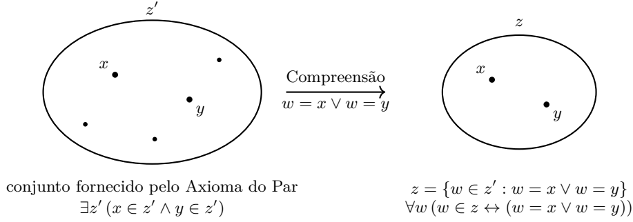
Figura 2.2: O Axioma do Par fornece um conjunto z' que possui x e y como elementos. Aplicando o Esquema da Compreensão a z' obtém-se o subconjunto z cujos únicos elementos são x e y .
