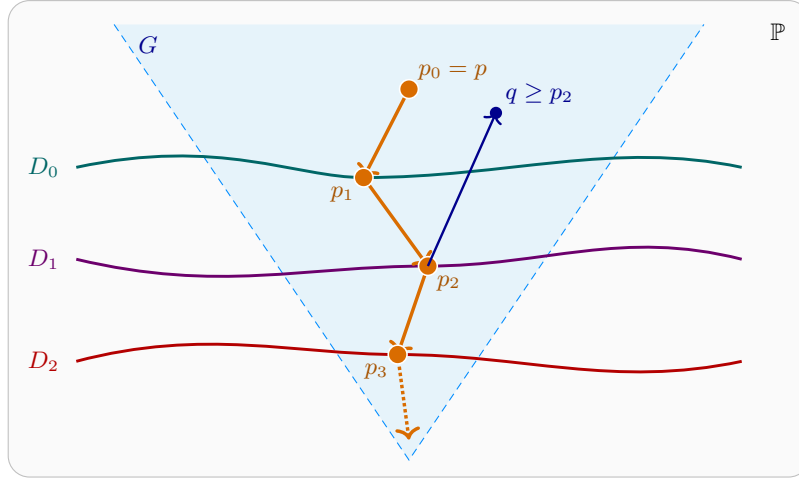
Figura 14.3: Ilustração da demonstração da Proposição 14.2.18.
