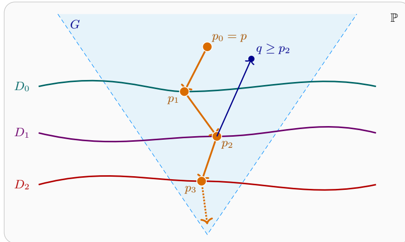
Figura 14.3: Ilustração da demonstração da Proposição 14.2.17.
