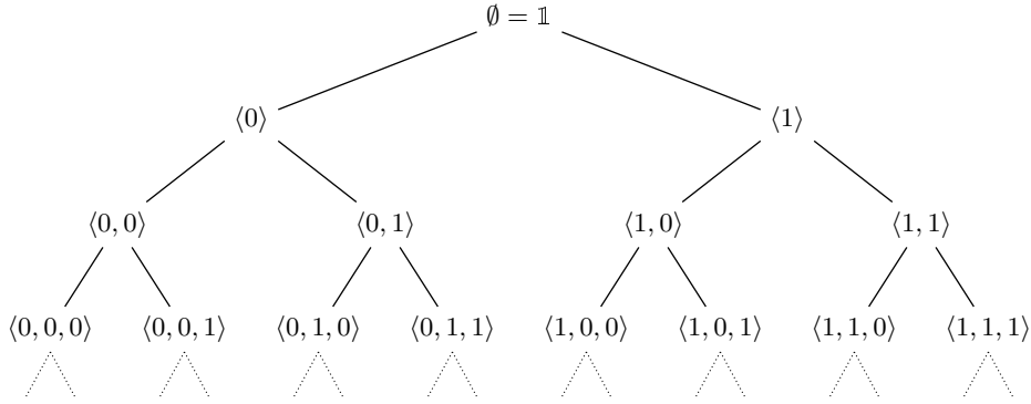
Figura 14.2: Os primeiros níveis de 2^{<\omega} .
