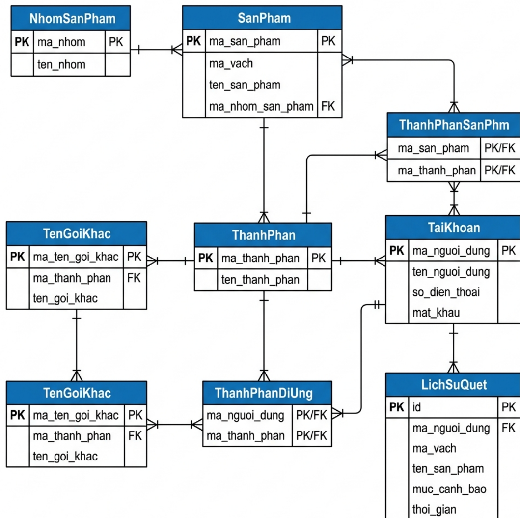
Hình 2.3: Sơ đồ ERD của cơ sở dữ liệu FOOD
