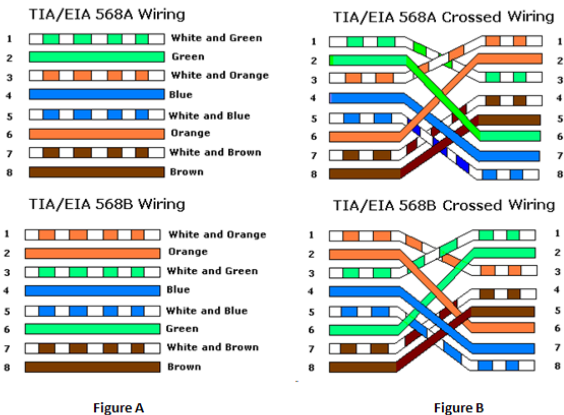
Obrázek 8: Přímé a křížené zapojení UTP kabelu
