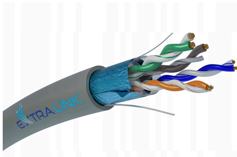
Obrázek 2: Kroucená dvoulinka (Twisted Pair)
