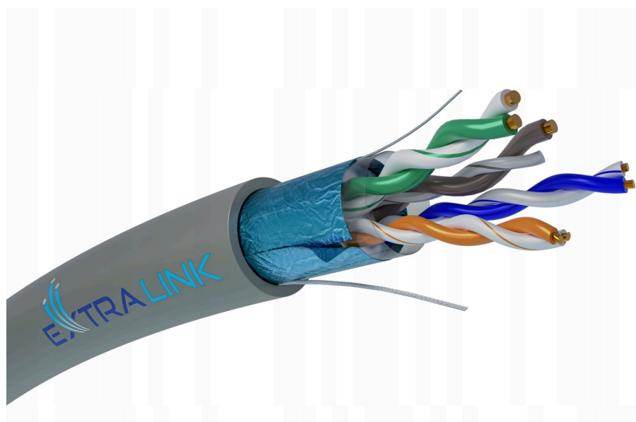
Obrázek 2: Kroucená dvoulinka (Twisted Pair)
