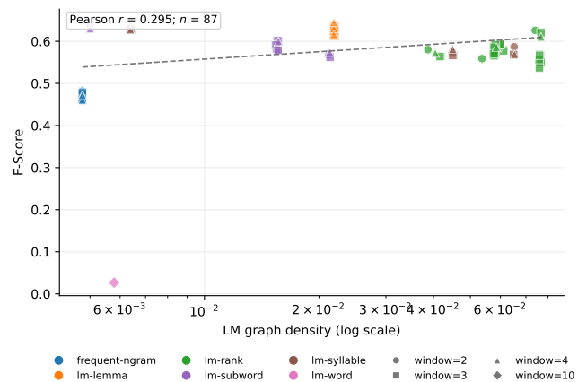
(d) POS—F-measure
