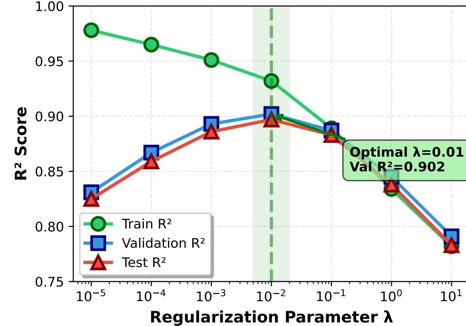
G. Regularization Parameter Tuning
