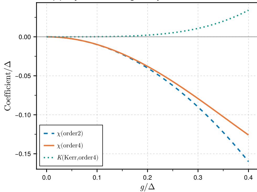
(d) Jaynes-Cummings: dispersive shift and Kerr
