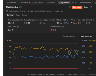
(b) 100 VUs.
