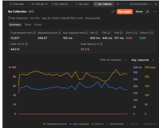
(a) 50 VUs.
