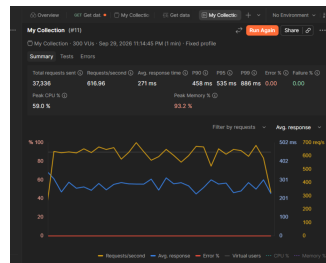
(d) 300 VUs.
