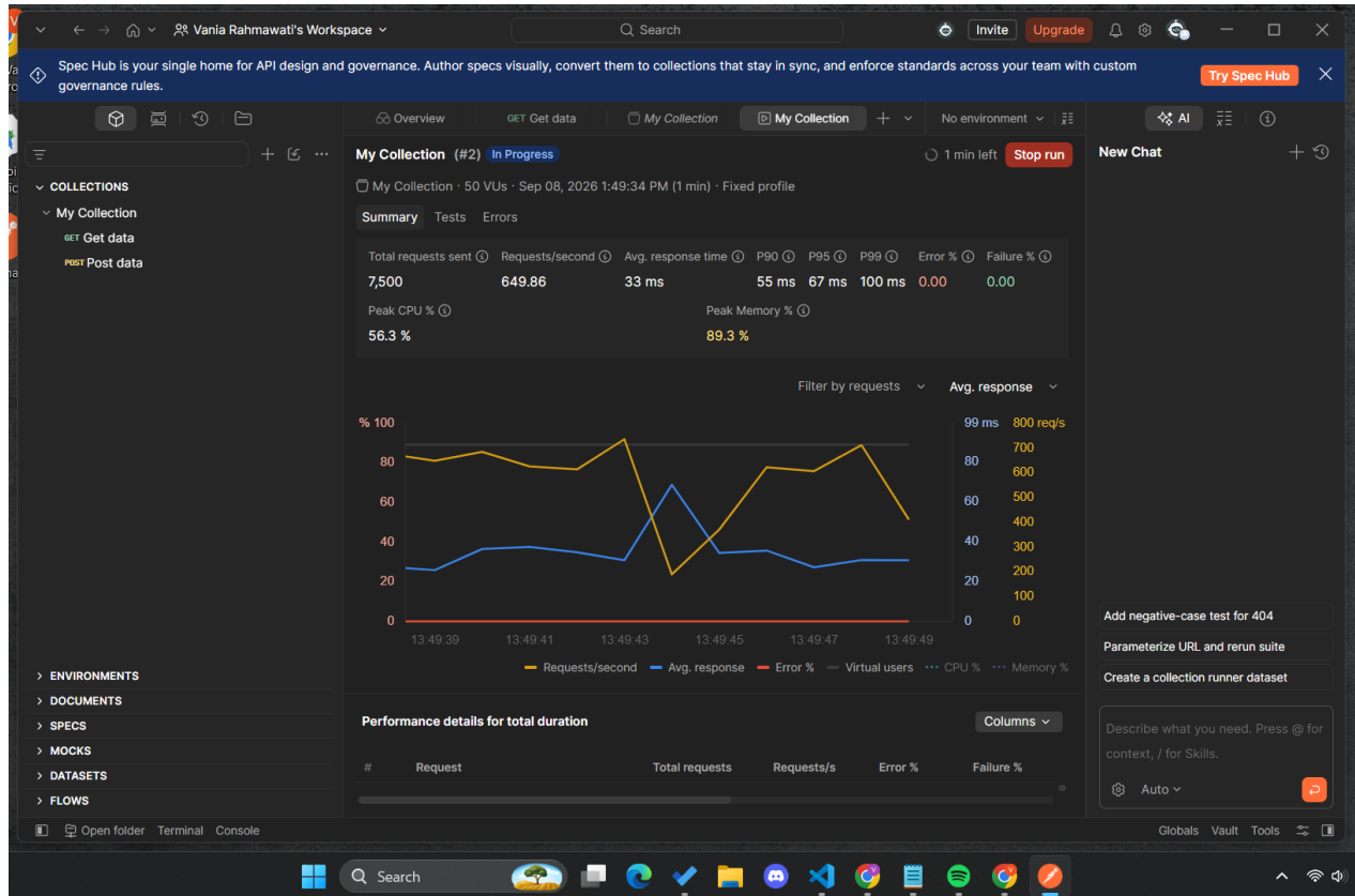
Fig. 12. Hasil Uji Beban 50 Pengguna dalam Semenit Menggunakan Postman.
