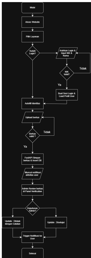
Fig. 10. Flowchart Pemohon Layanan.
