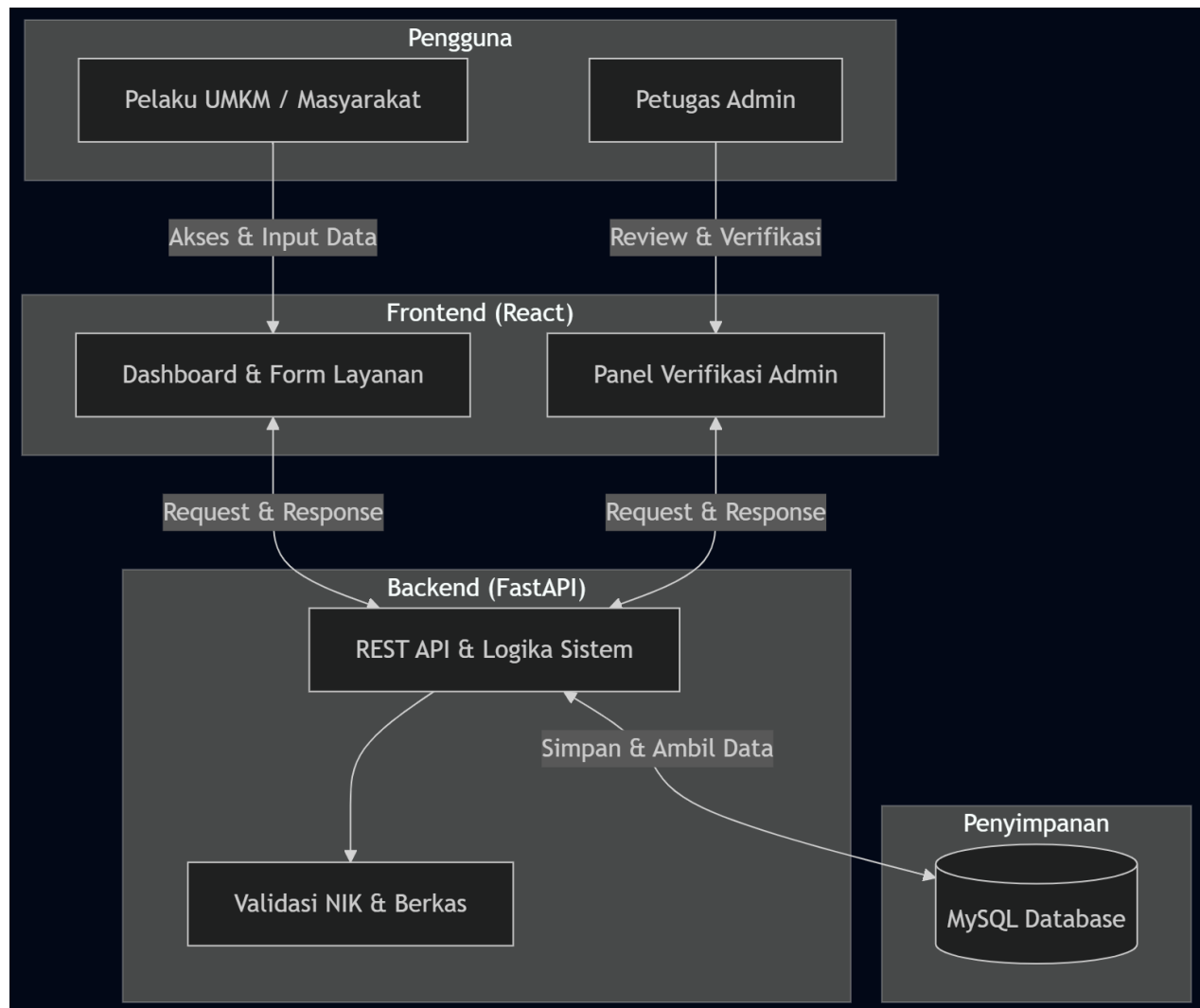
Fig. 2. Desain Arsitektur Sistem SI-UMKM Jabar.
