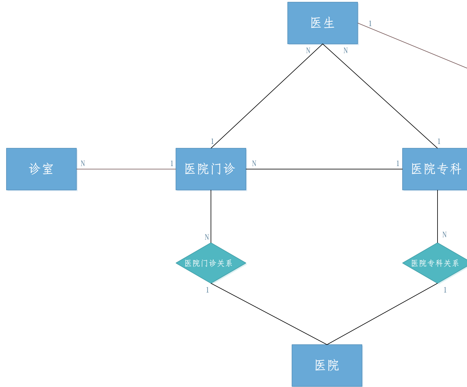
挂号通ER图-医院部分
