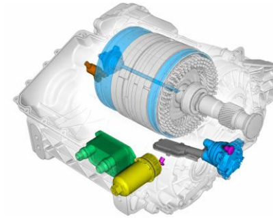
후륜 전기 모터 오일 냉각 시스템
