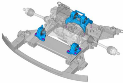
전륜 전기 모터 마운팅 대형 부싱
