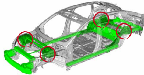
앞 뒤 스프링 스트럿 타워 고압 다이캐스팅 알루미늄 적용
