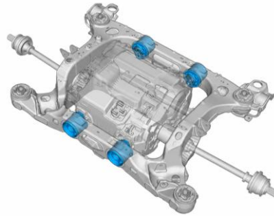
후륜 전기 모터 마운팅 대형 부싱
