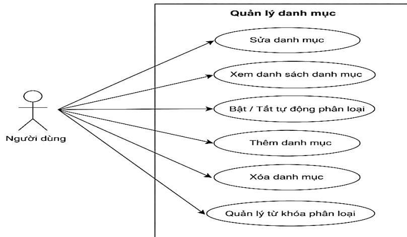
Hình 5: Use case quản lý danh mục
