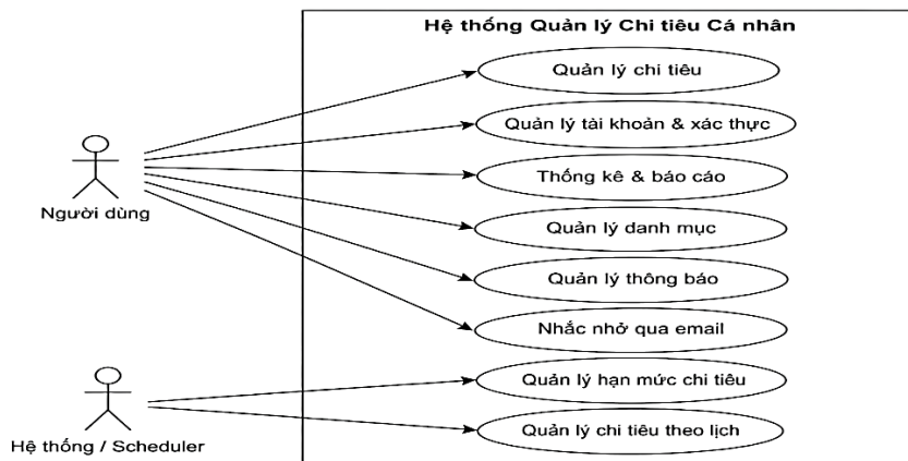
Hình 3: Sơ đồ use case tổng quát
