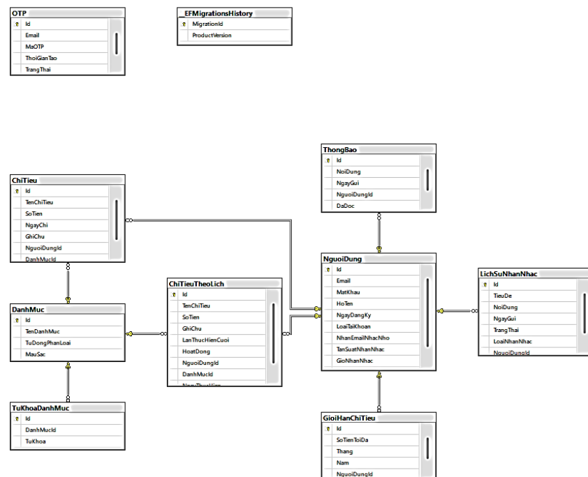
Hình 1: Lược đồ cơ sở dữ liệu
