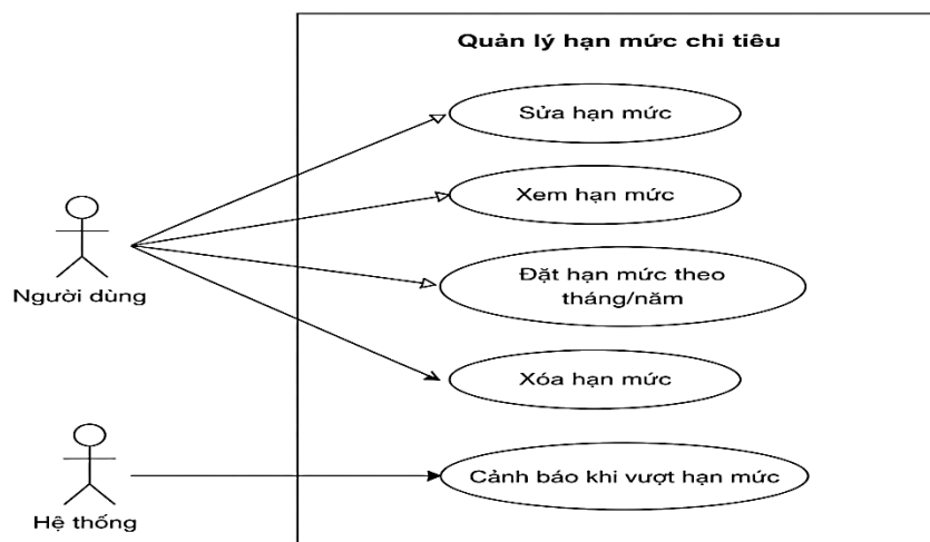
Hình 10: Use case quản lý hạn mức chi tiêu
