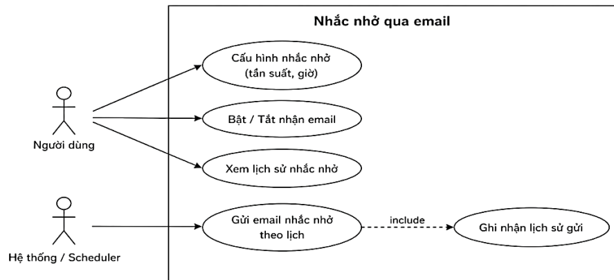
Hình 13: Use case quản lý nhắc nhở
