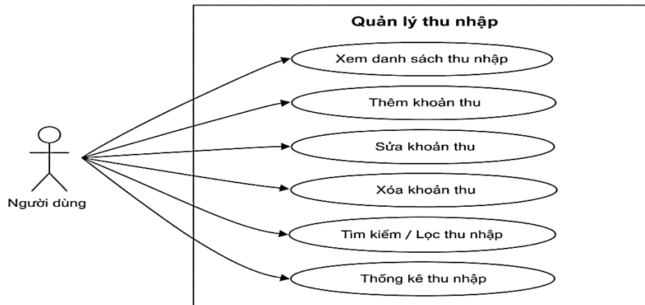
Hình 7: Use case quản lý thu nhập
