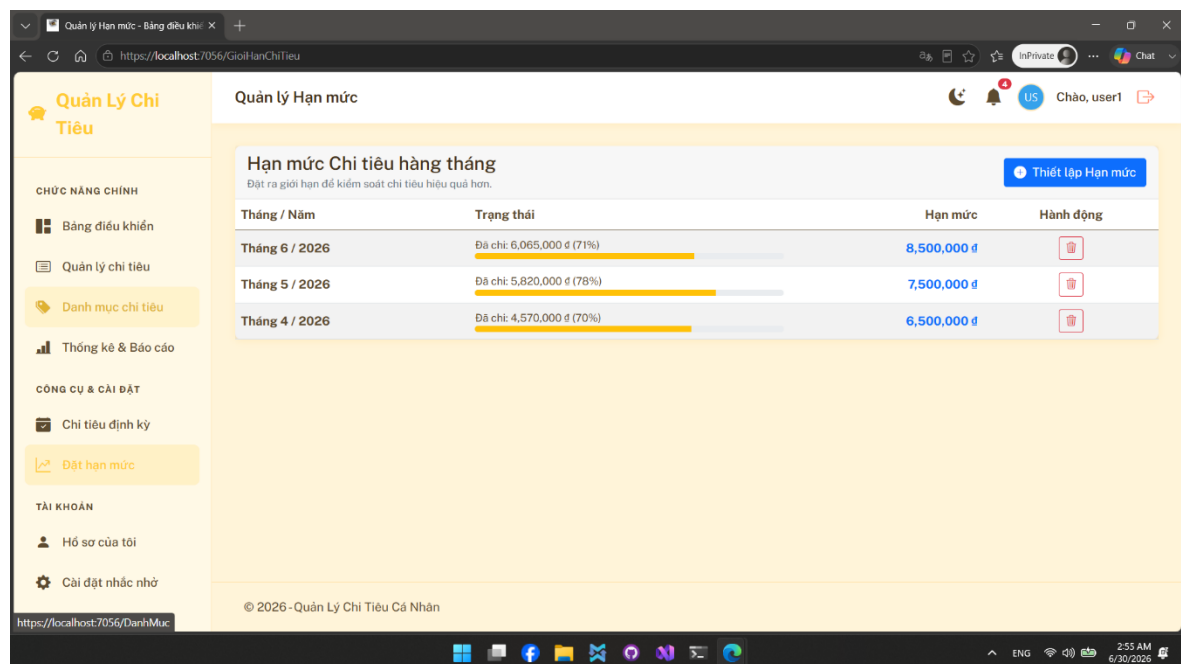
Hình 27: Giao diện đặt hạn mức chi tiêu
