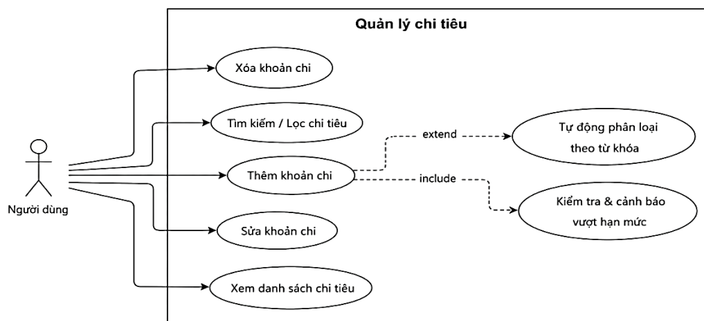
Hình 6: Use case quản lý chi tiêu
