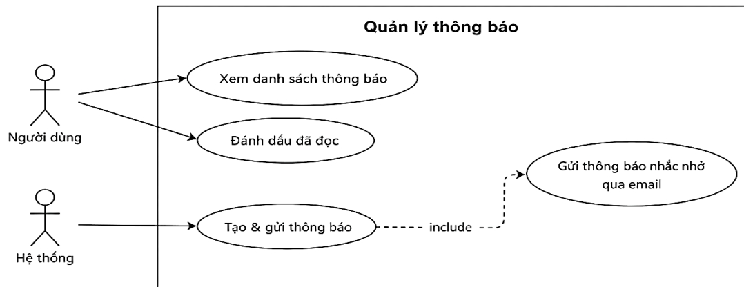
Hình 12: Use case quản lý thông báo
