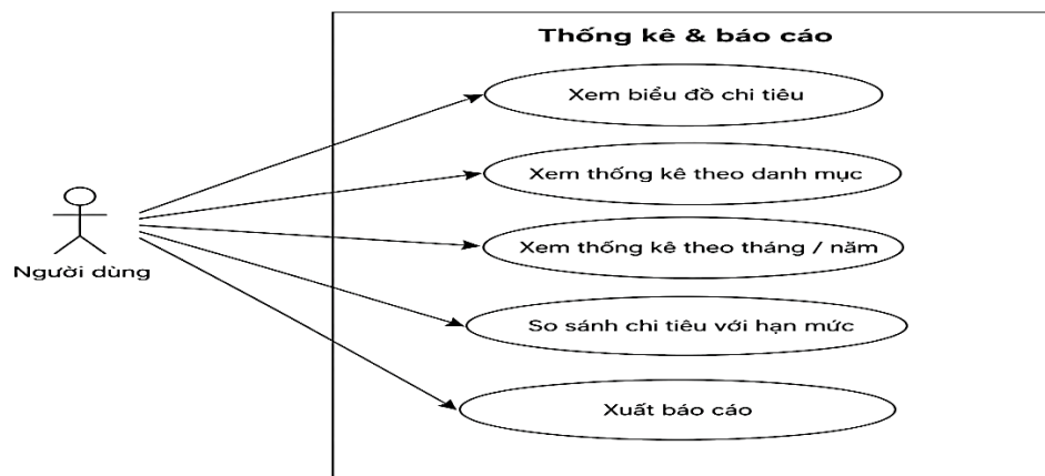
Hình 11: Use case thống kê và báo cáo
