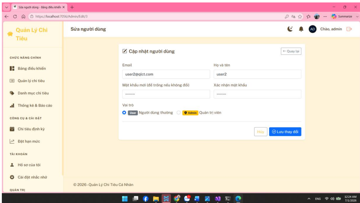
Hình 33: Giao diện chỉnh sửa người dùng (Admin)
