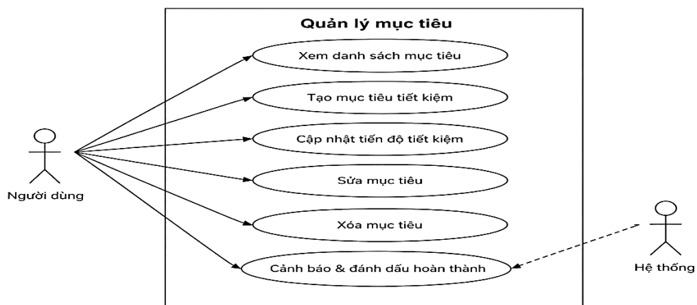
Hình 8: Use case quản lý mục tiêu
