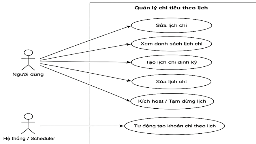
Hình 9: Use case quản lý chi tiêu theo lịch
