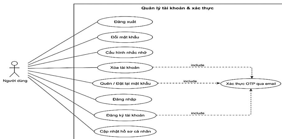
Hình 4: Use case quản lý tài khoản & xác thực
