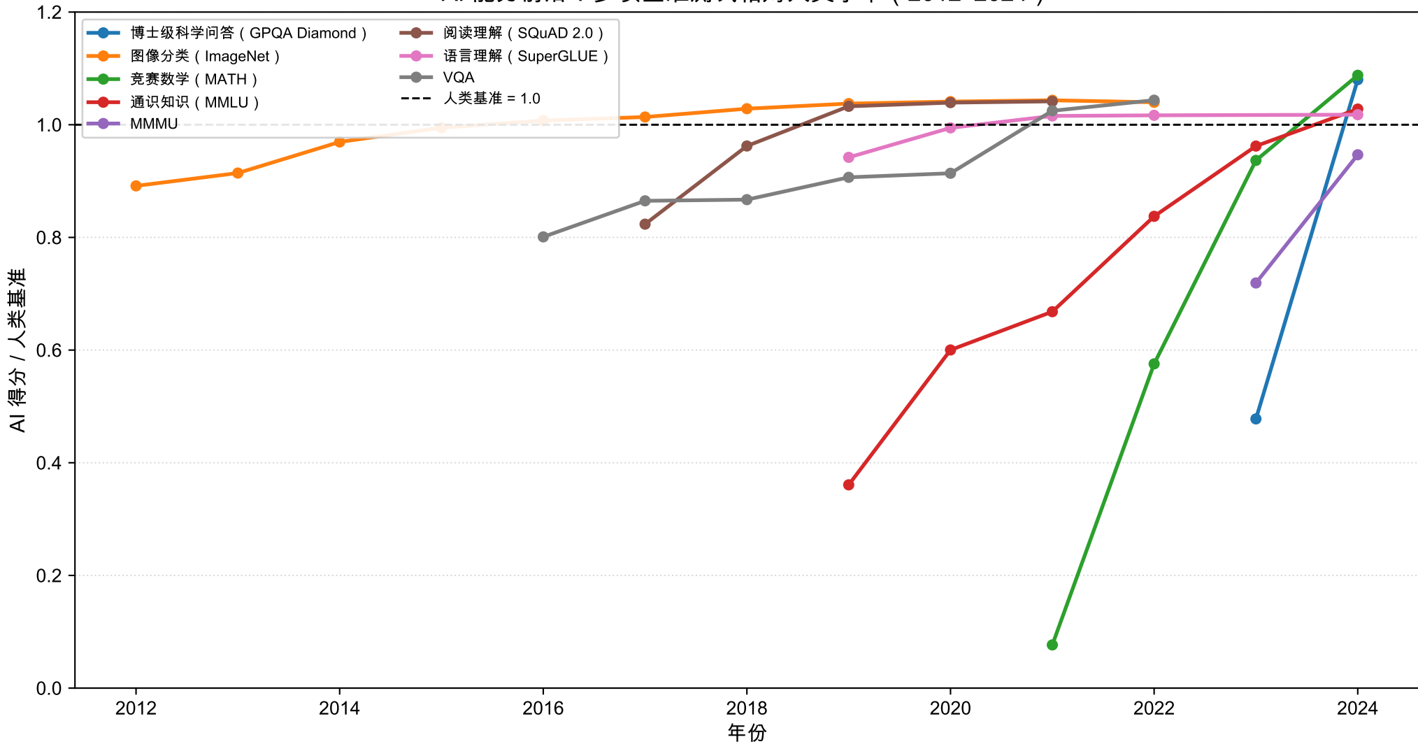
AI 能力前沿：多项基准测试相对人类水平 ( 2012–2024 )
