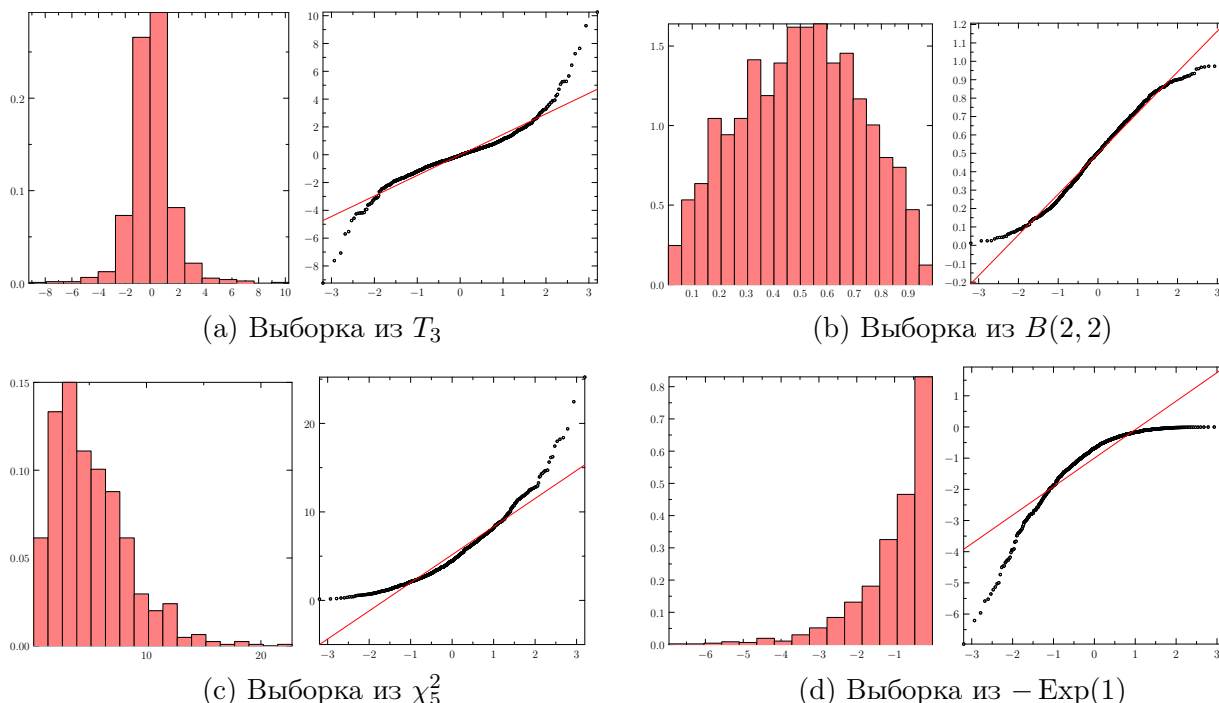
Рис. 3: Normal QQ-plot для различных распределений
