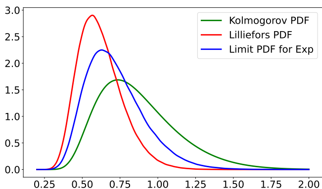
Рис. 4: Плотности предельных распределений
