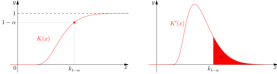
Рис. 1: CDF и PDF распределения Колмогорова
