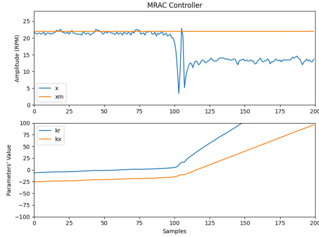
Διάγραμμα 4.3.1 Drift παραμέτρων.
