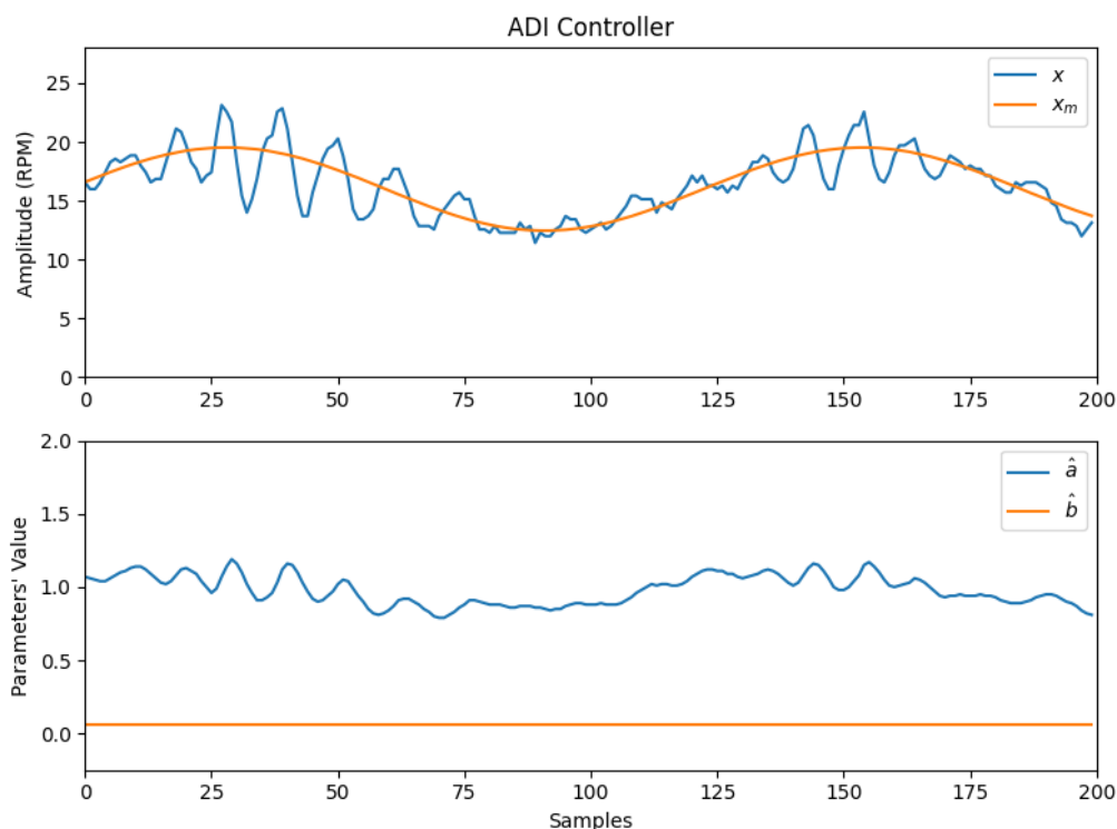
Διάγραμμα 5.2.1 Παρακολούθηση του ημιτονοειδούς σήματος αναφοράς και έλεγχος των .
